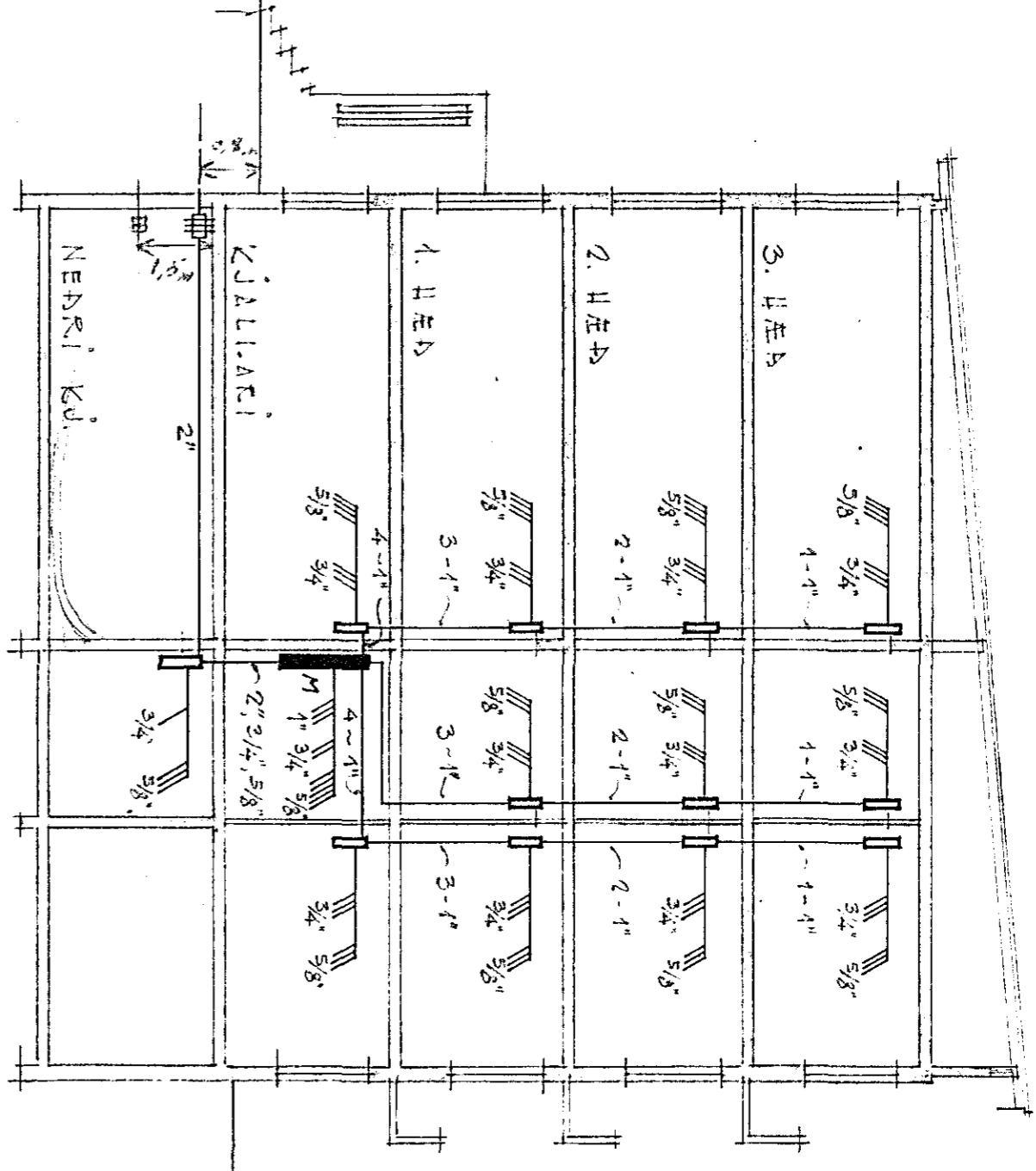
SNEIÐIN 1 M = 1:100
