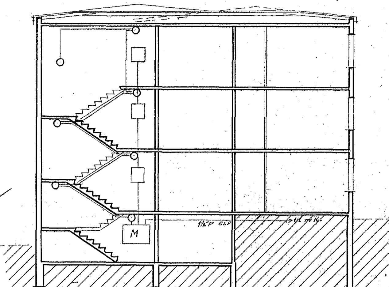
SKURÐUR
