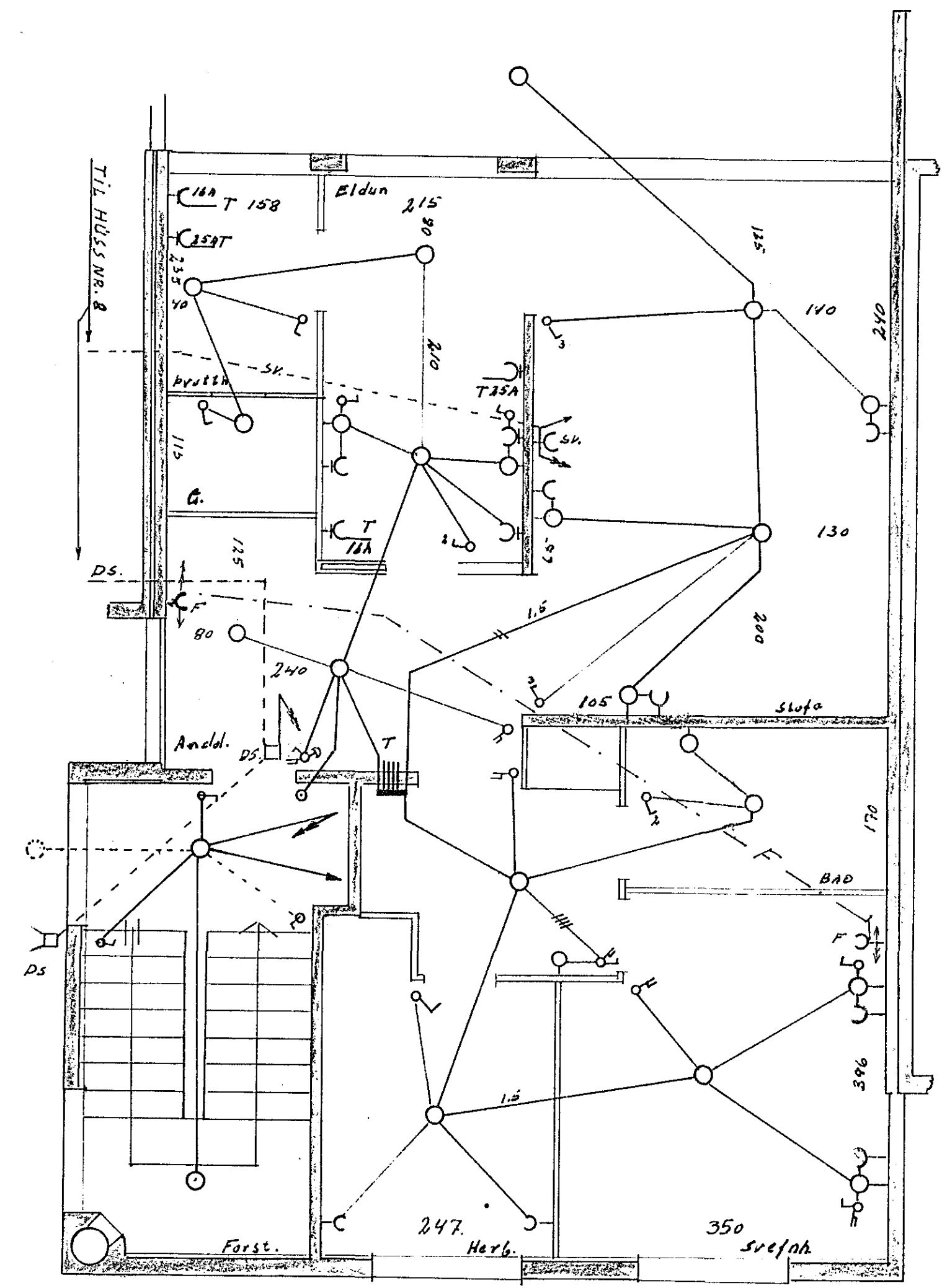
1. og 3. Hæð
