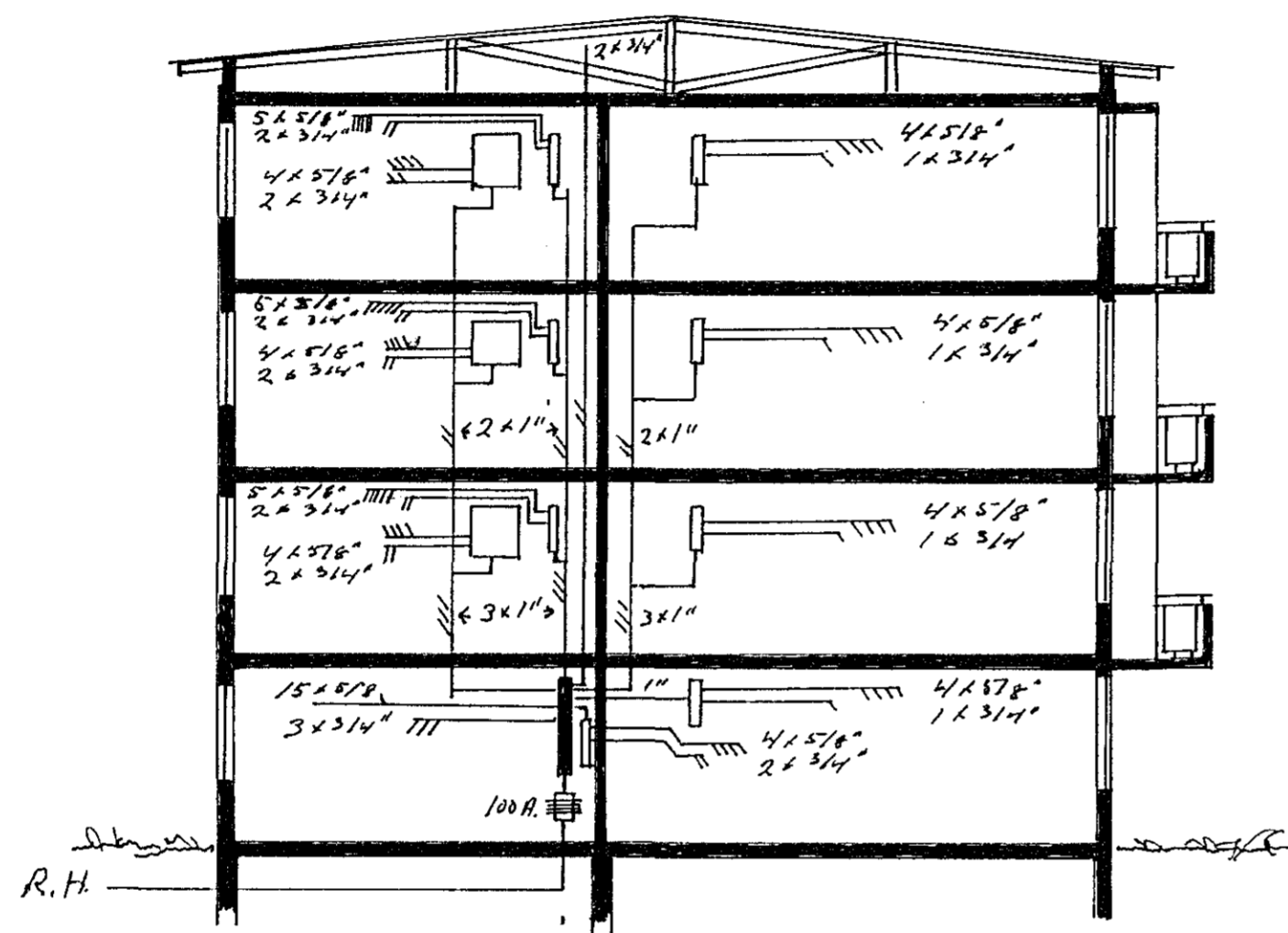
SKURÐUR
