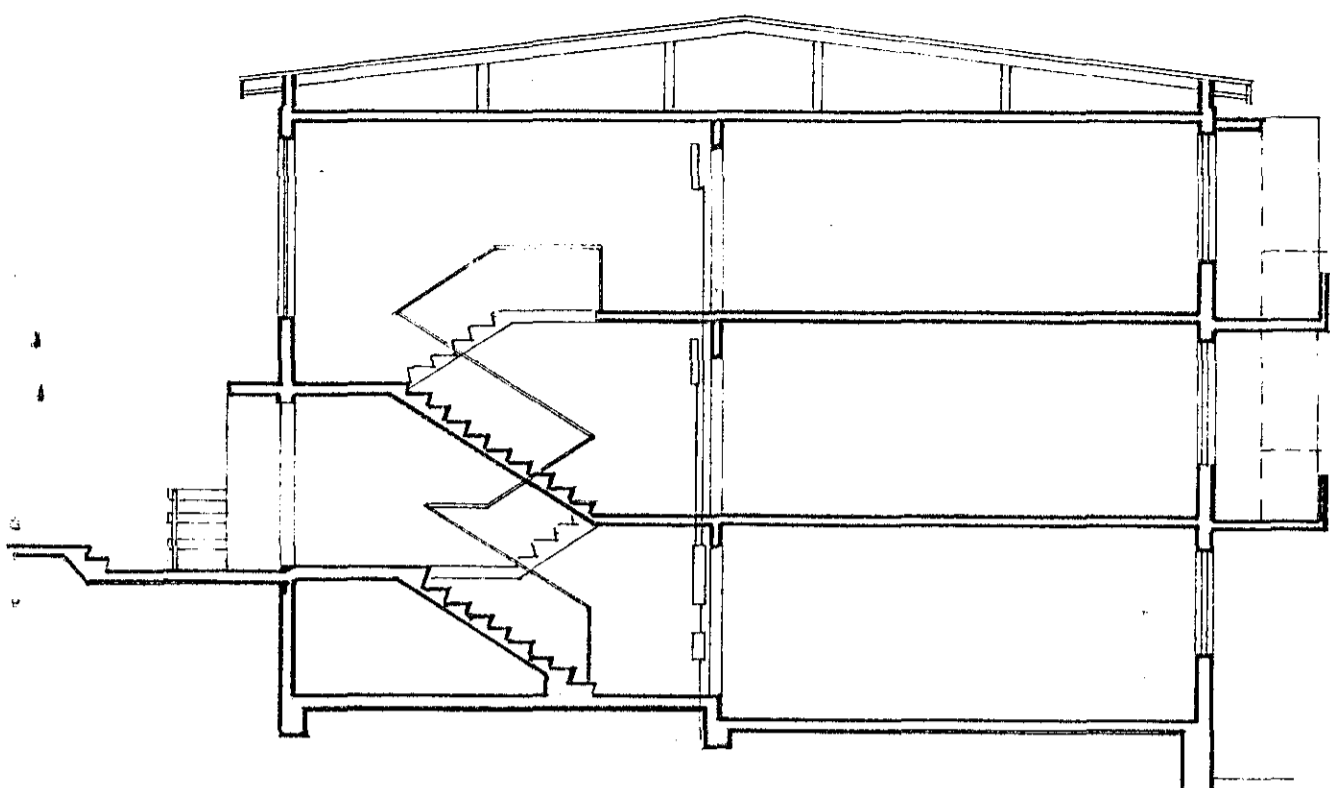
Snið M. 1:100
