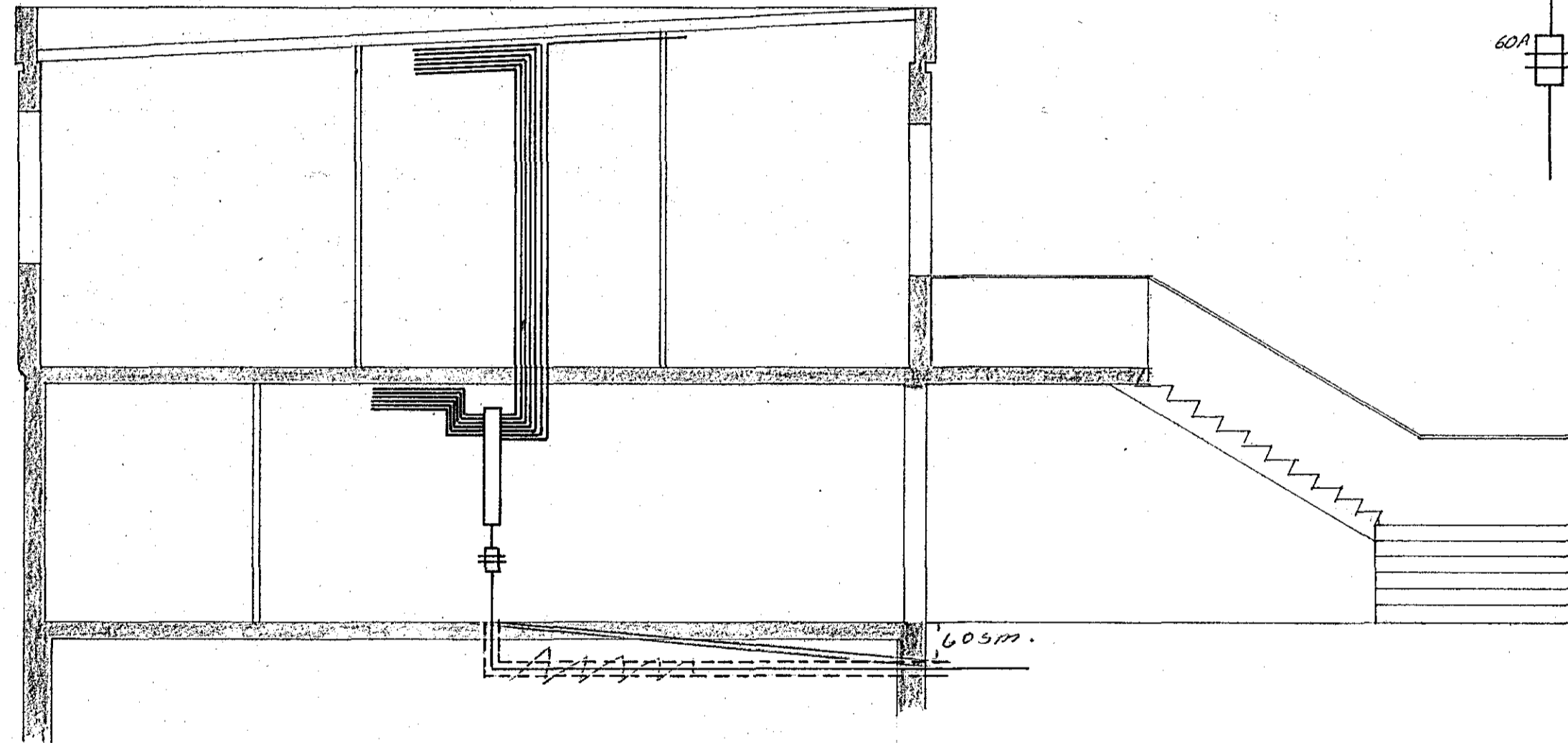
Þverskurður
