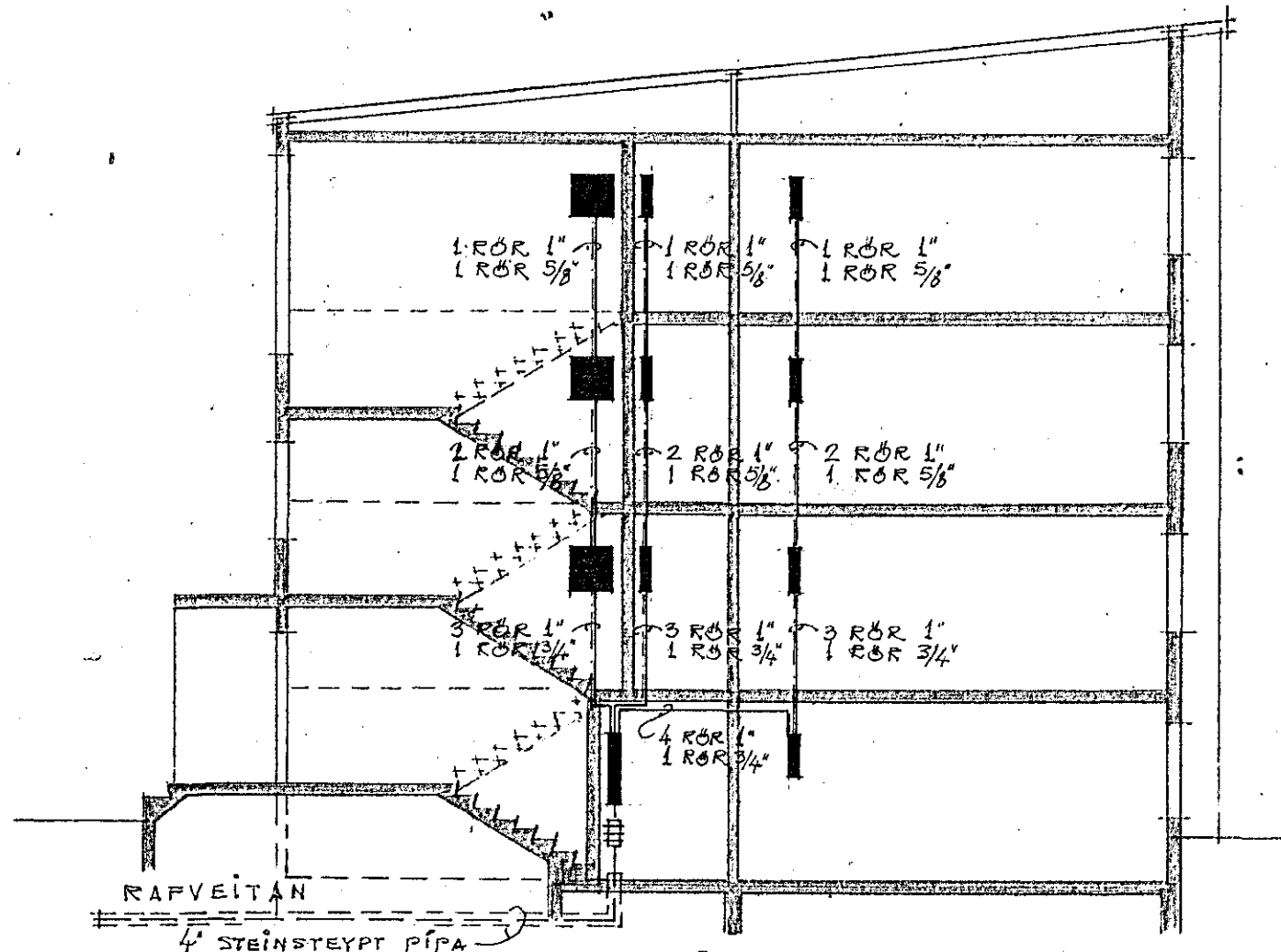
SNEIÐING "B"
