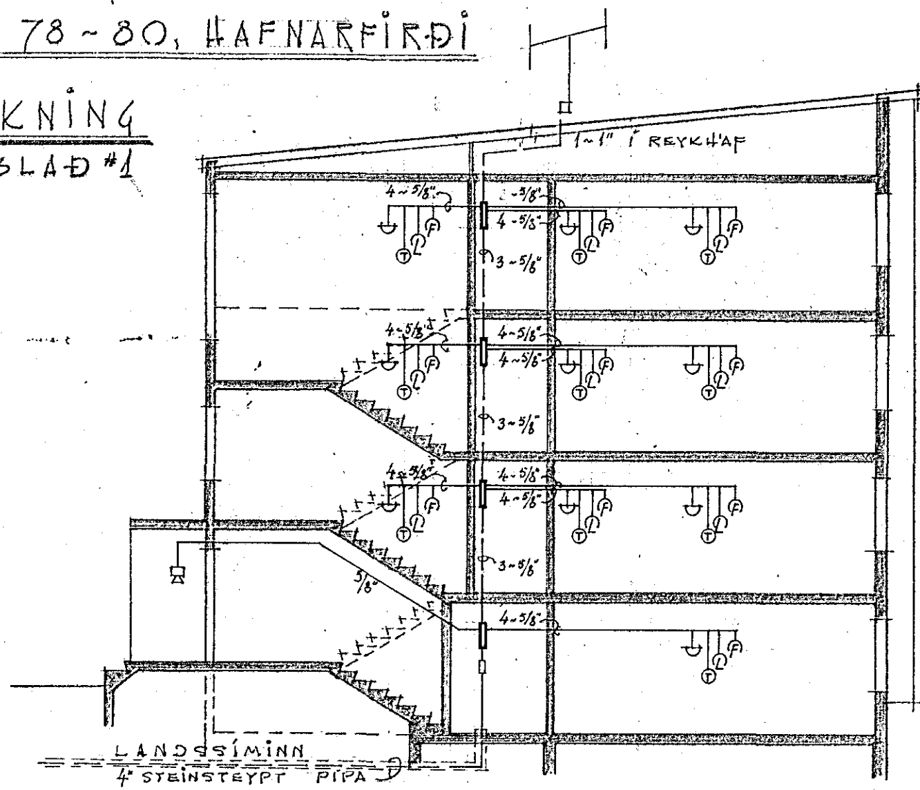
SNEIÐING "A"
