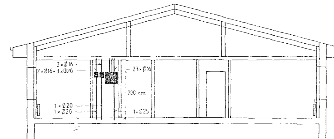
Snið A-A
