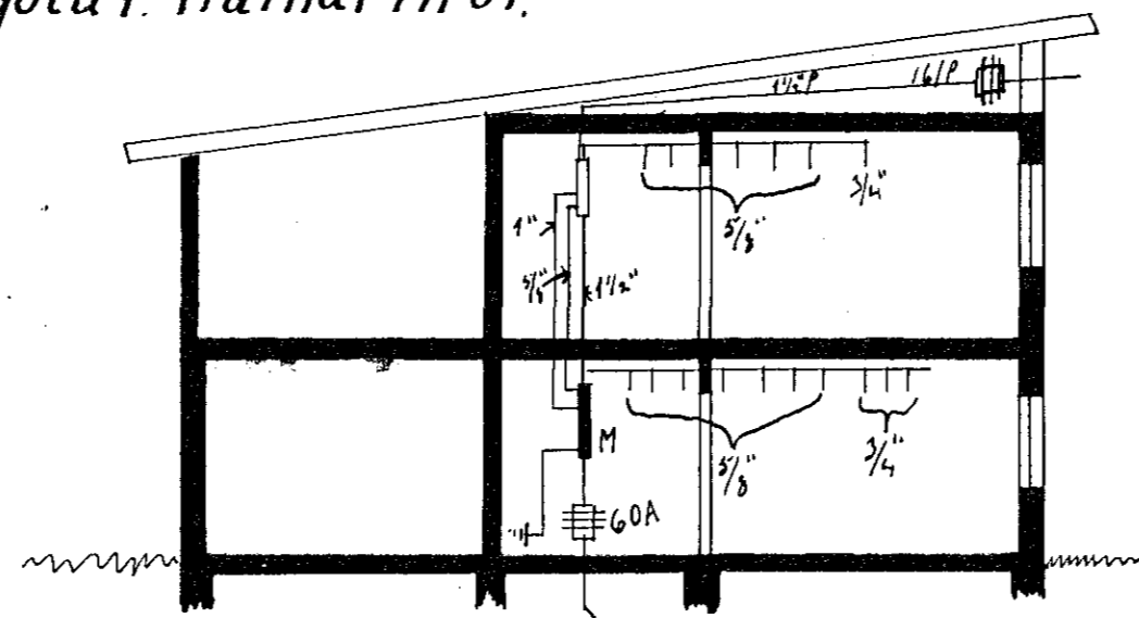
ÞVERSKURÐUR
