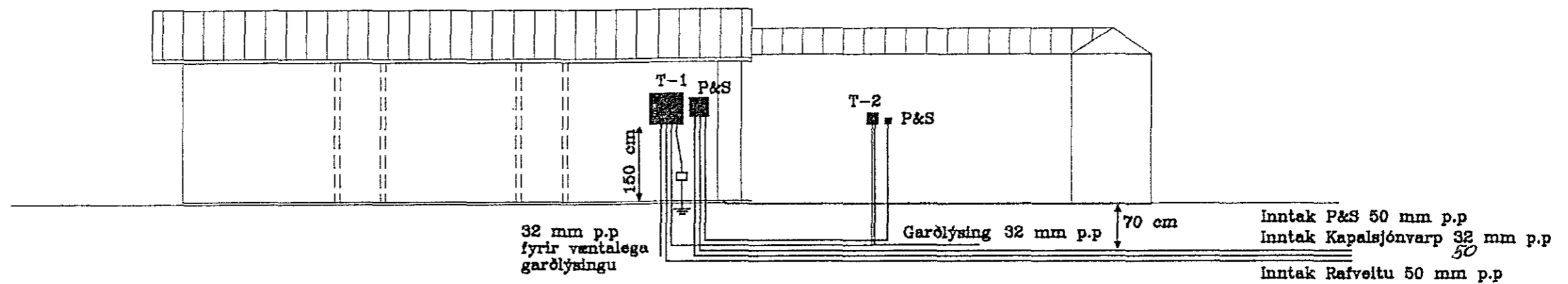
Austurhlið snið A - A
