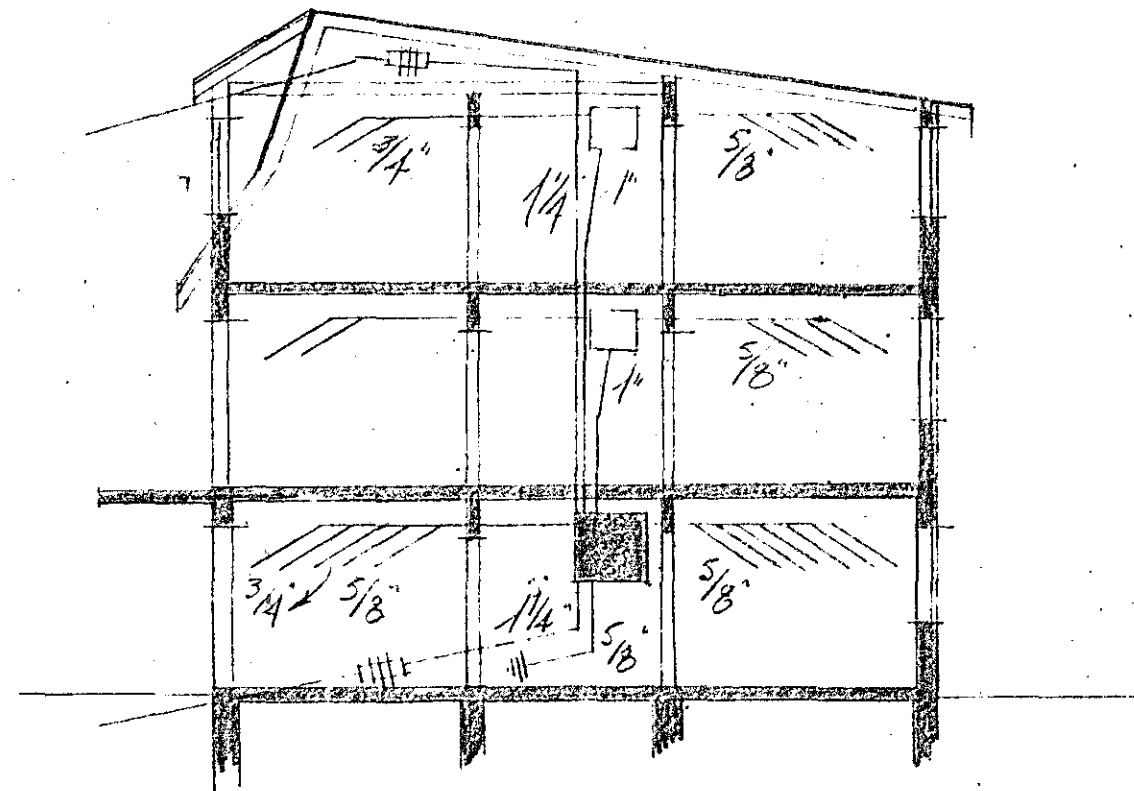
SKURÐUR.
