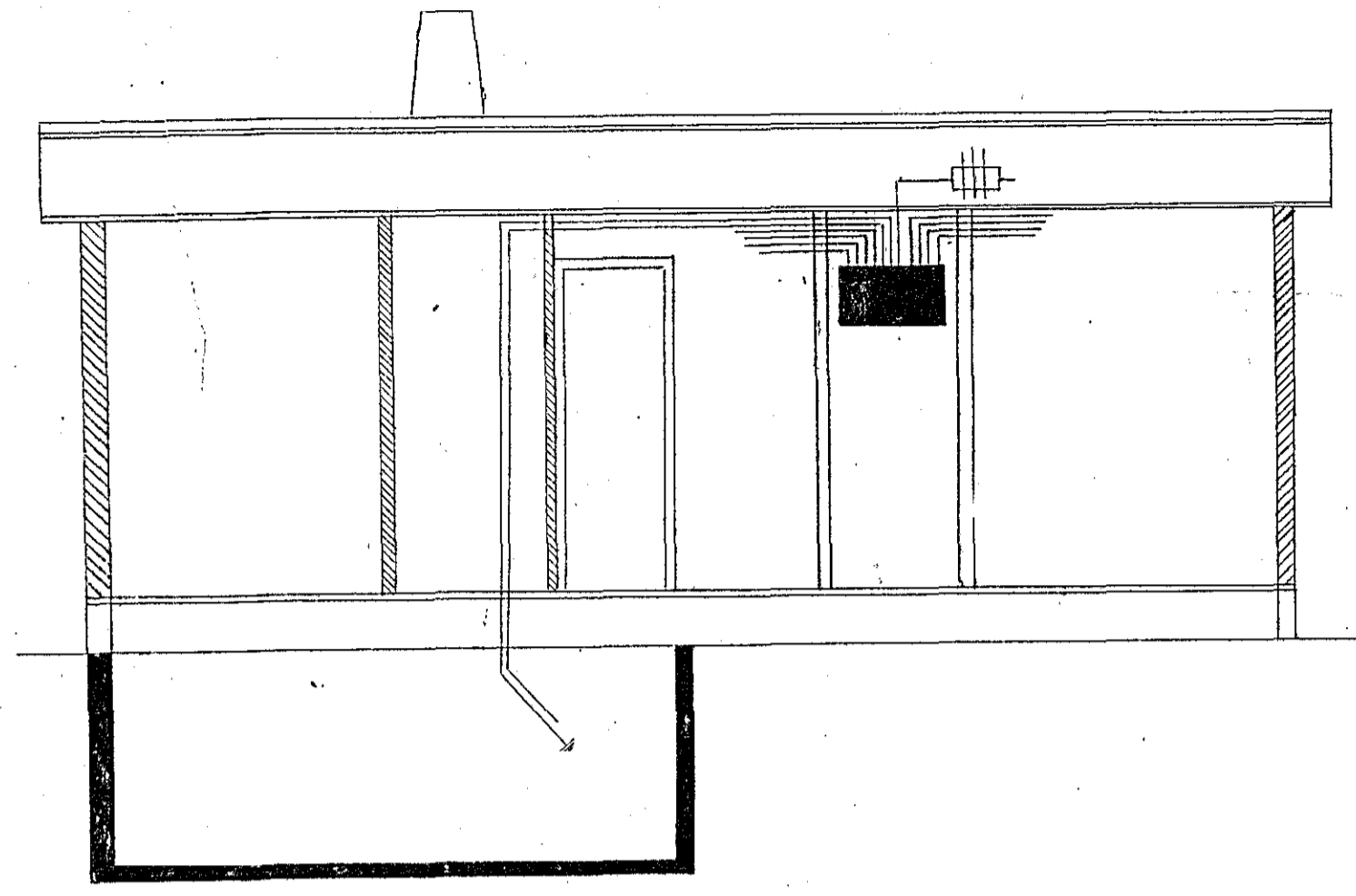
SKURÐUR.
