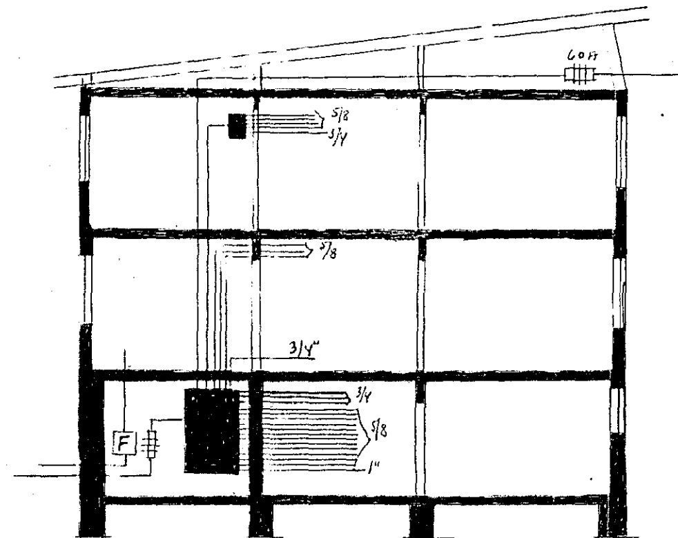
Skurður
