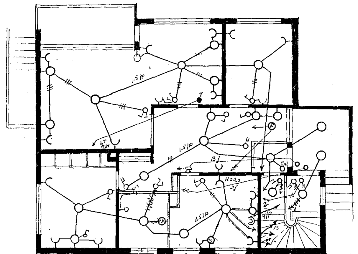
1. Hæð
