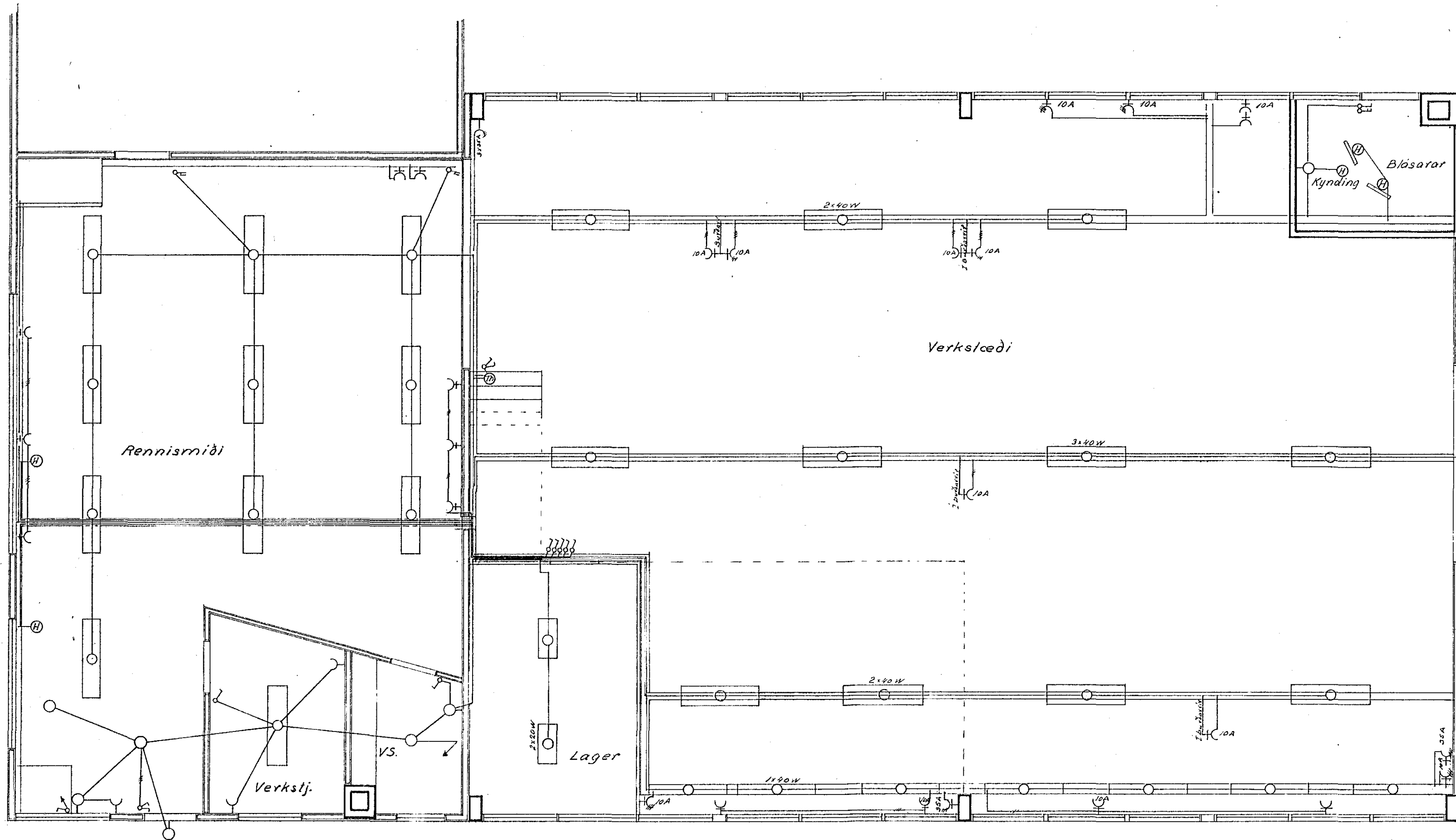
Grunnmynd I.hæðar
