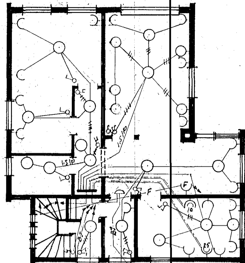
1. HÆÐ
