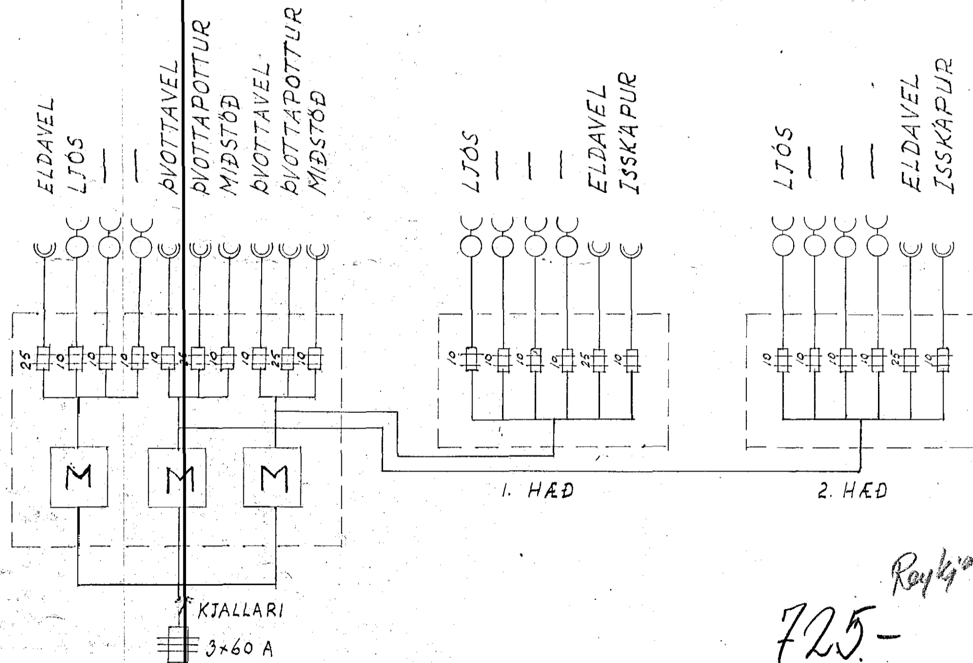
1. HÆÐ
