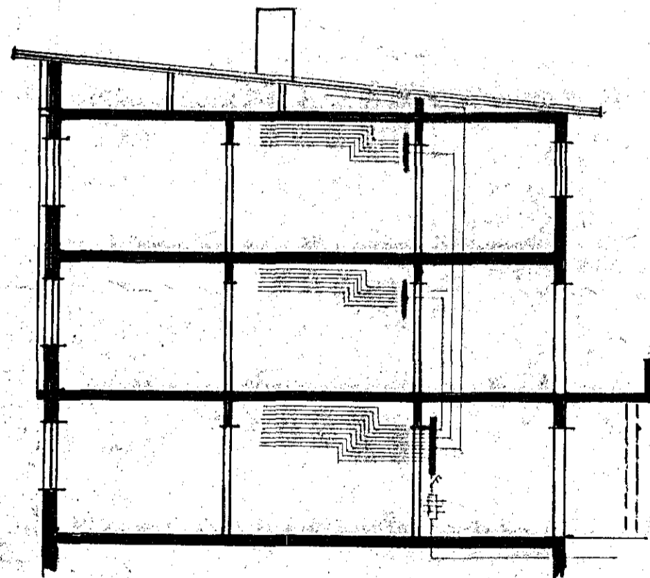
SKURÐUR
