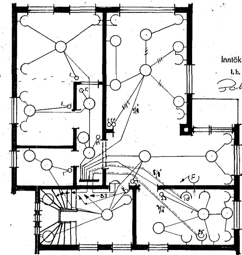
2. HÆÐ
