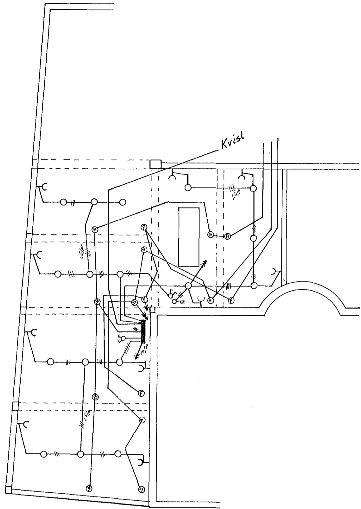
Kjallari m 1:100
