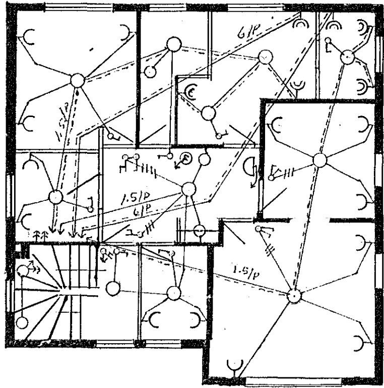
Þak hæð
