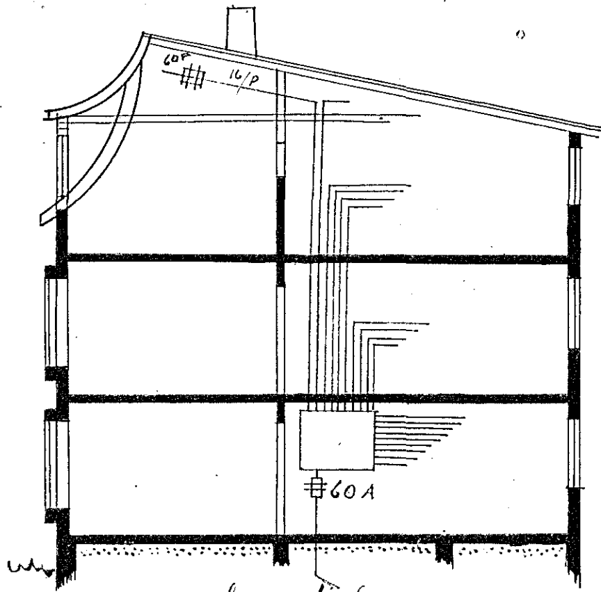
Þverskurður
