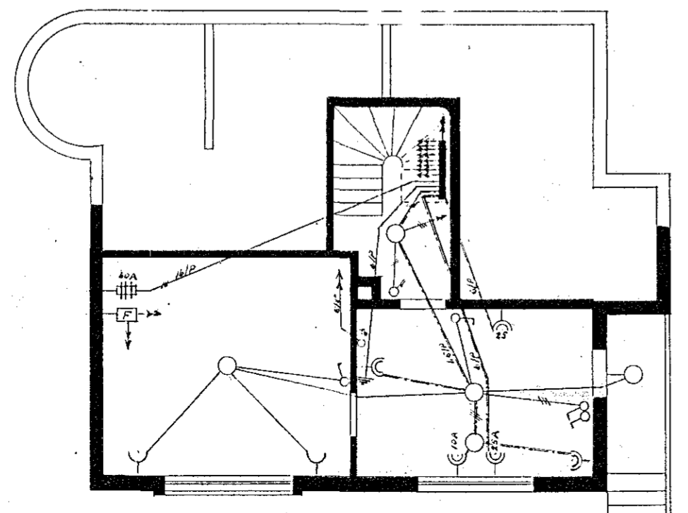
Kjallari
