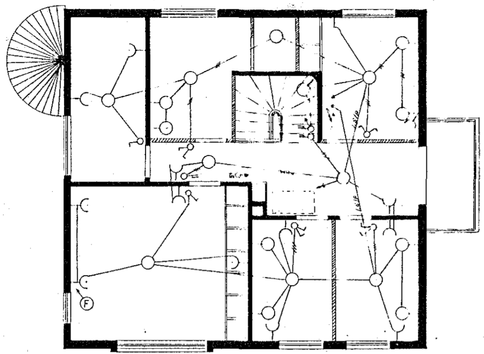
II. Hæð
