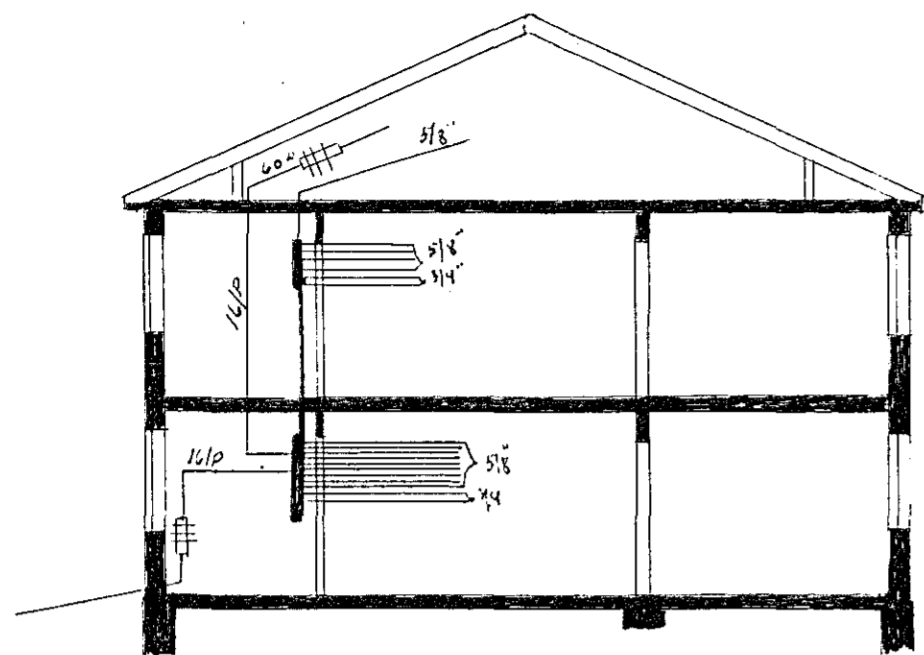
Skurður
