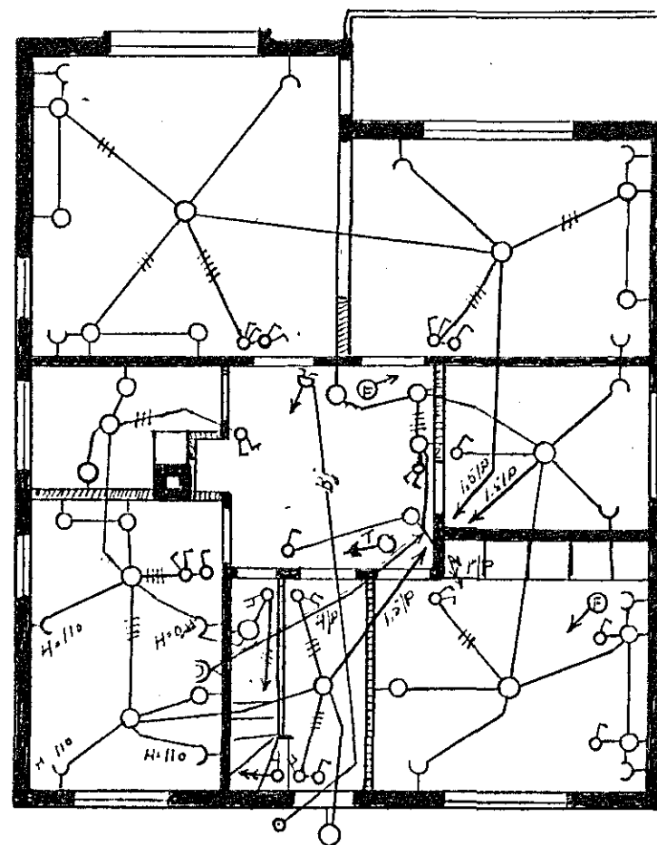
II. hæð
