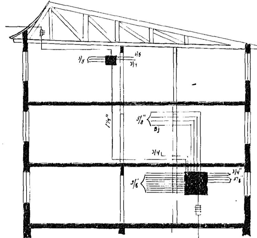
Skurður
