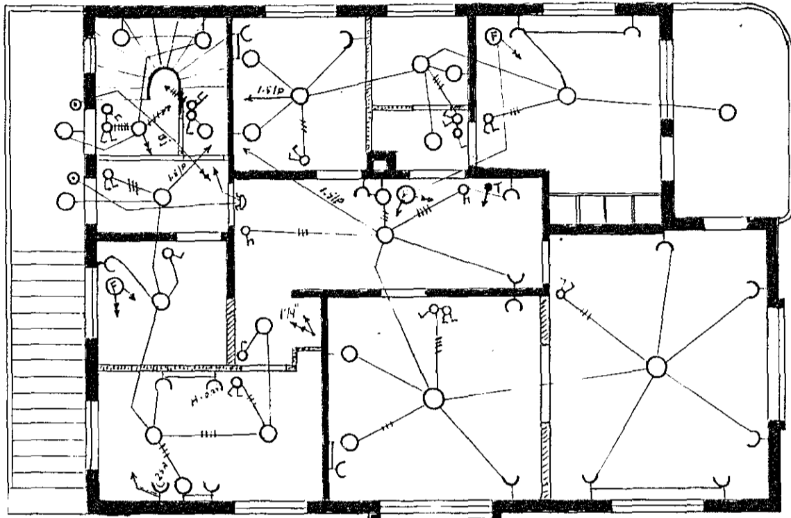
I. Hæð.
