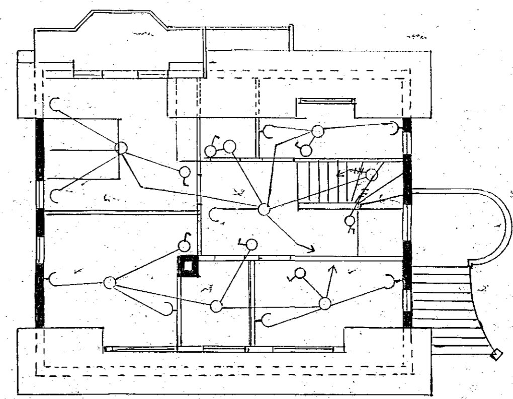
2. HÆÐ.
