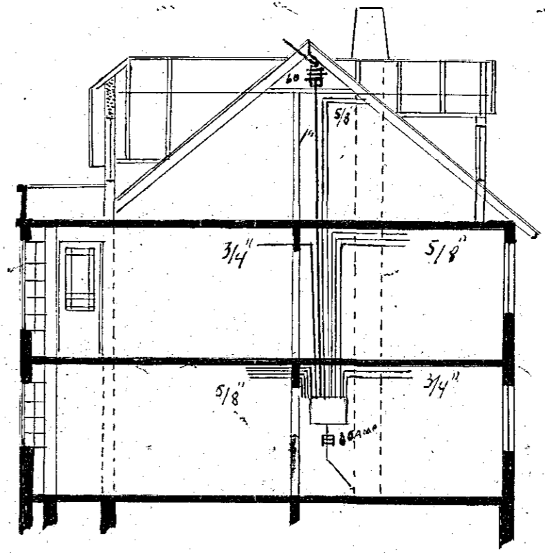
ÞVERSKURÐUR.
