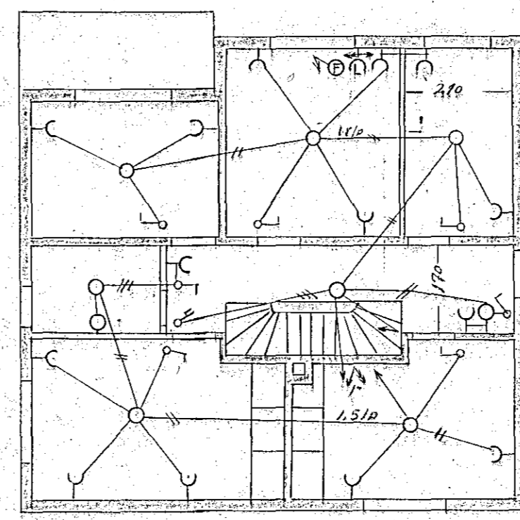
2. hæð
