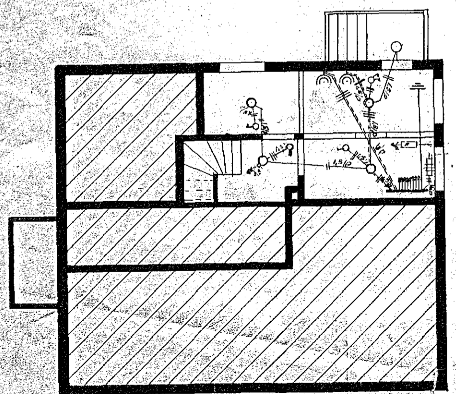
Kjallari
