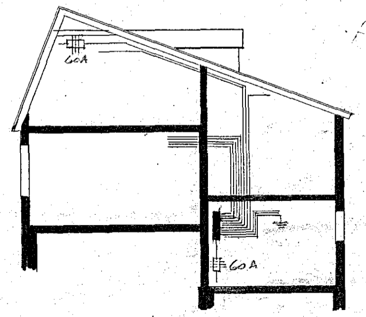
Þverskurður 397
