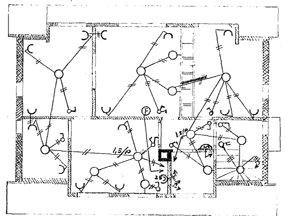
Risthæð.
