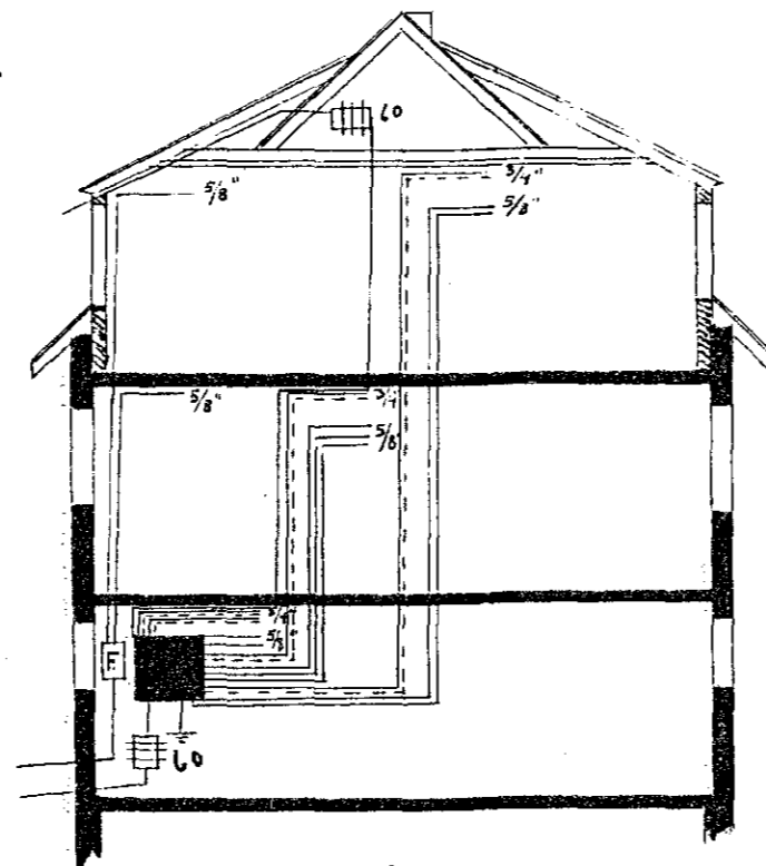
sneið.
