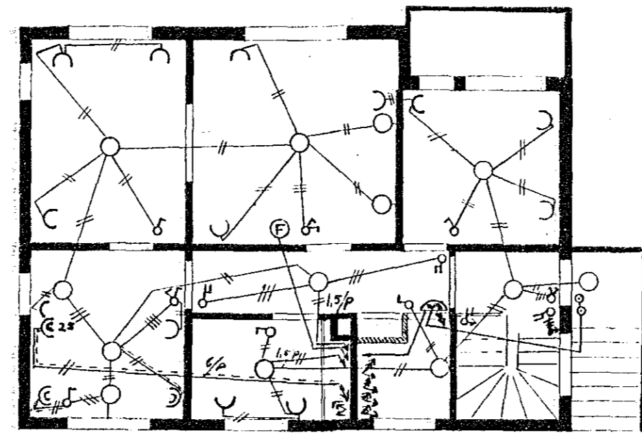
I. hæð.
