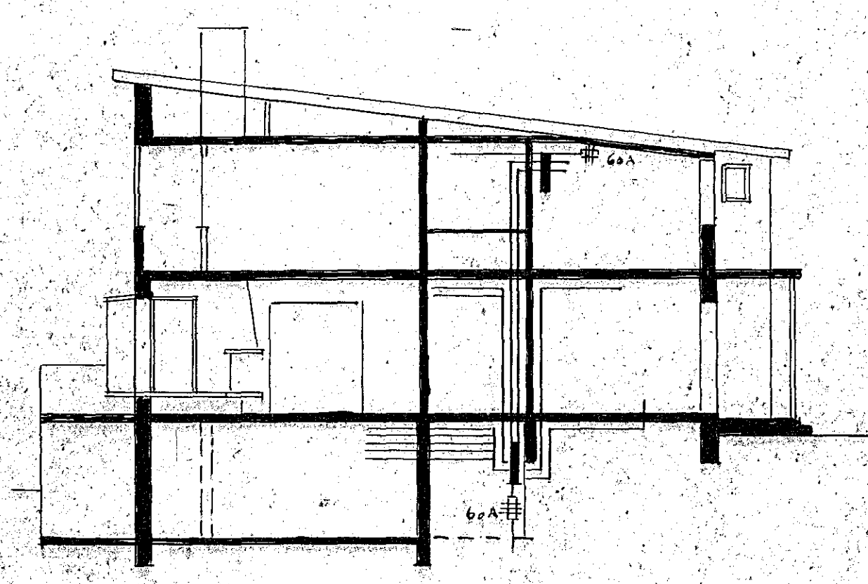
Sneiðing
