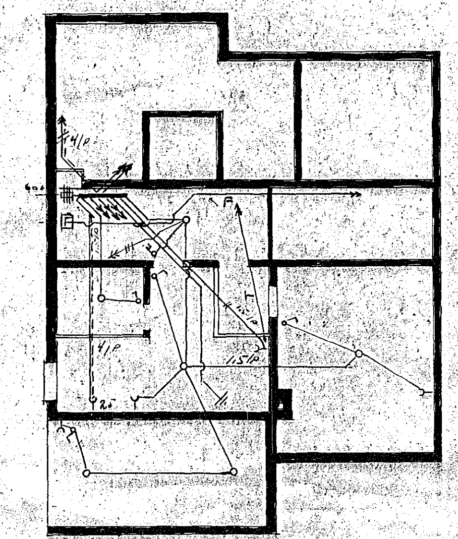
Grunnmynd
