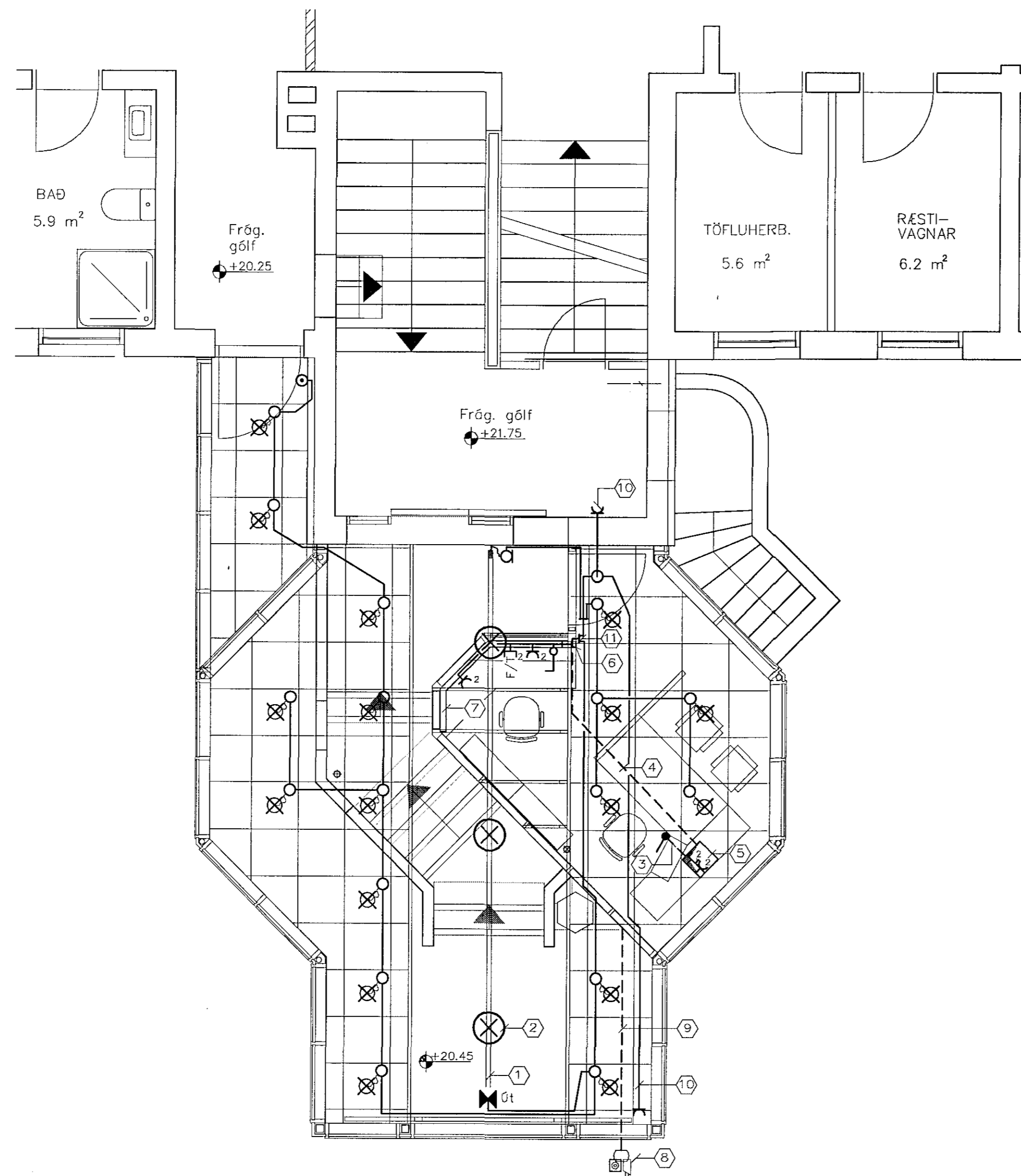
GRUNNMYND - RAFLÖGN 1:50
