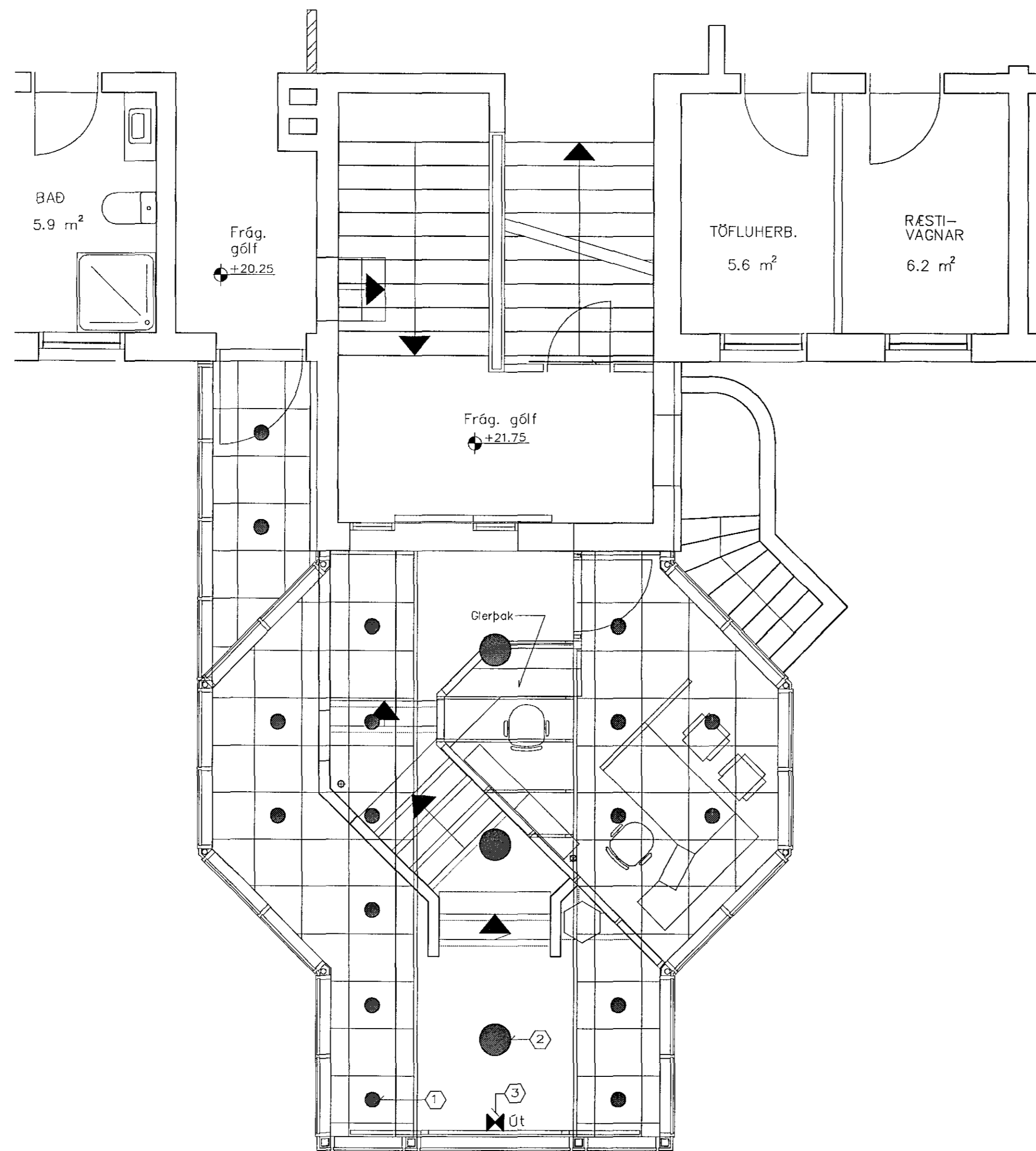
GRUNNMYND – LAMPAPLAN 1:50
