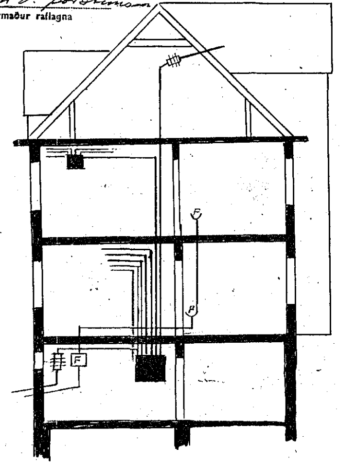
þverskurður
