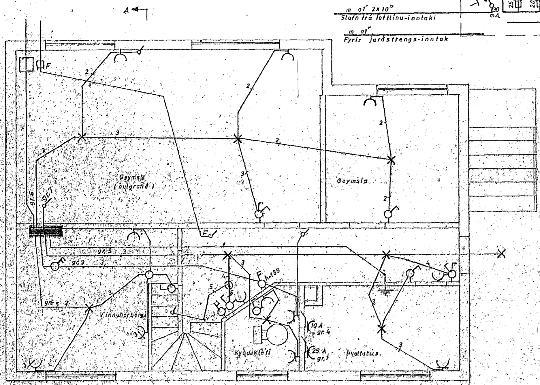
KJALLARI
