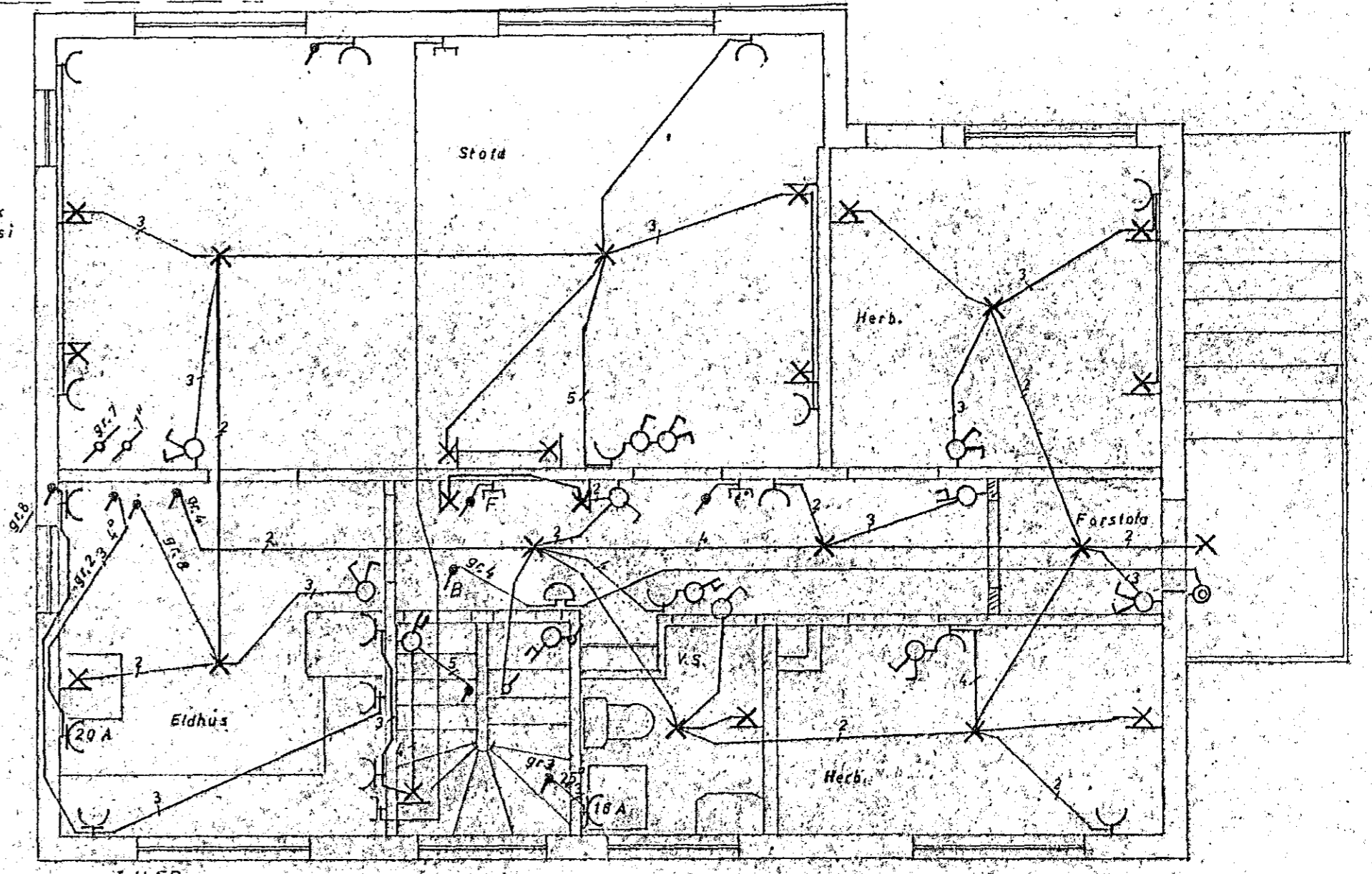
I.HÆÐ
