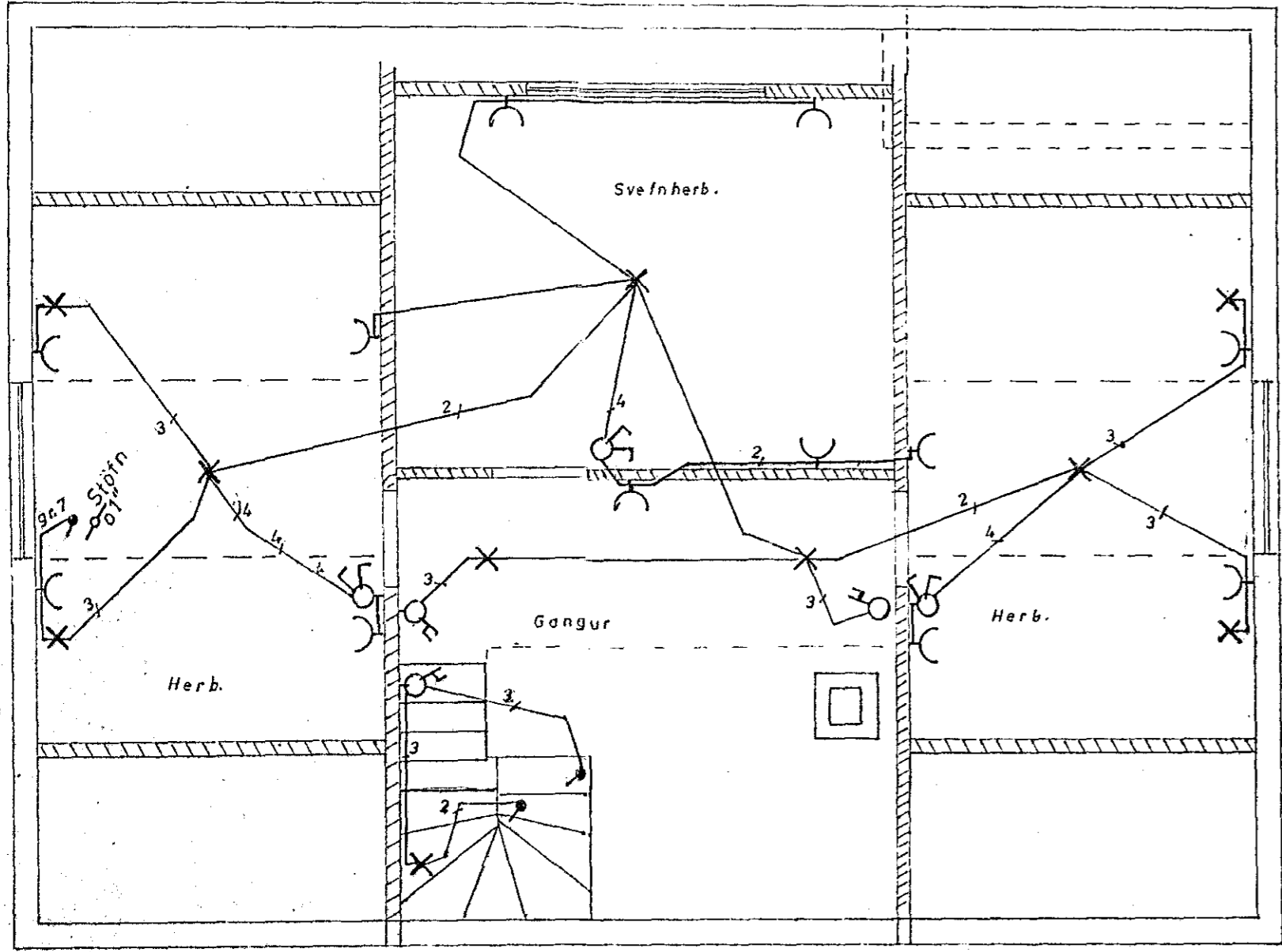
II.HÆÐ (RIS)
