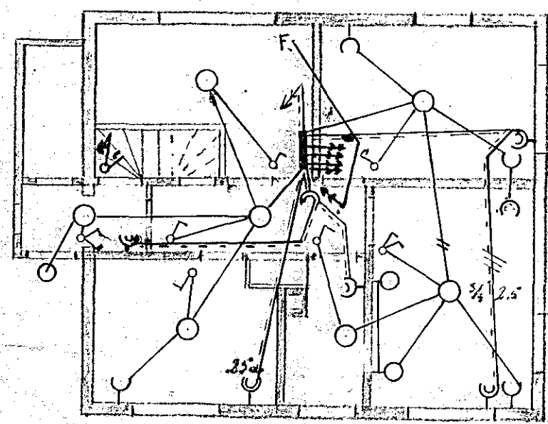
Kjallari
