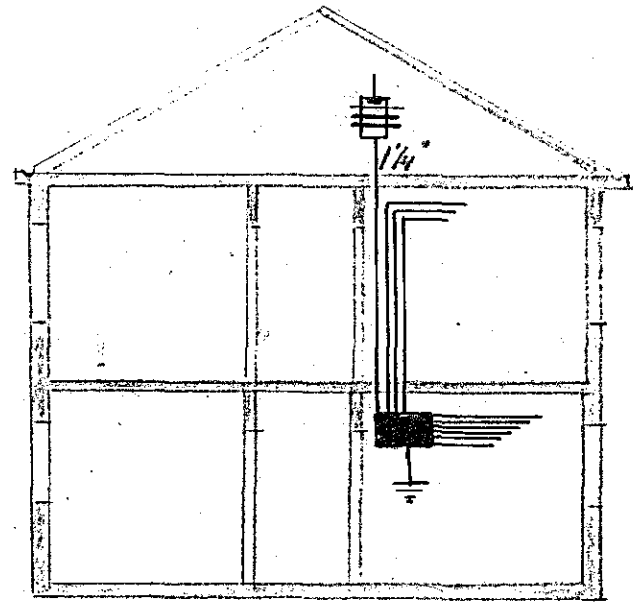
Sneiðing.
