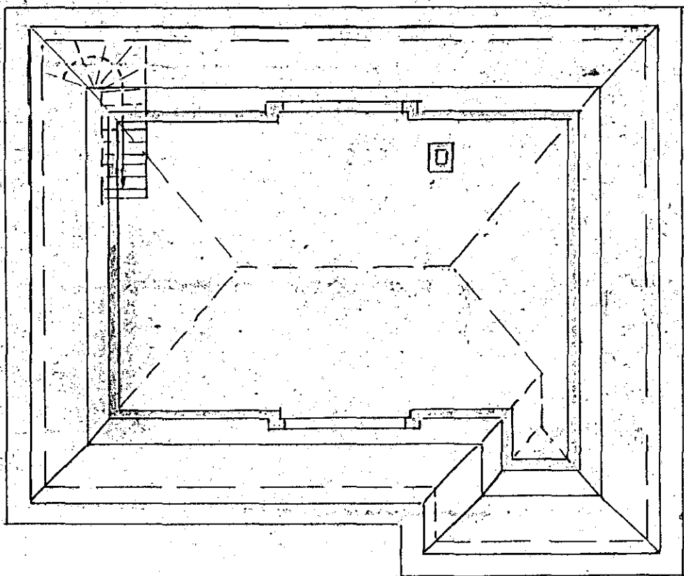
Rishæð
