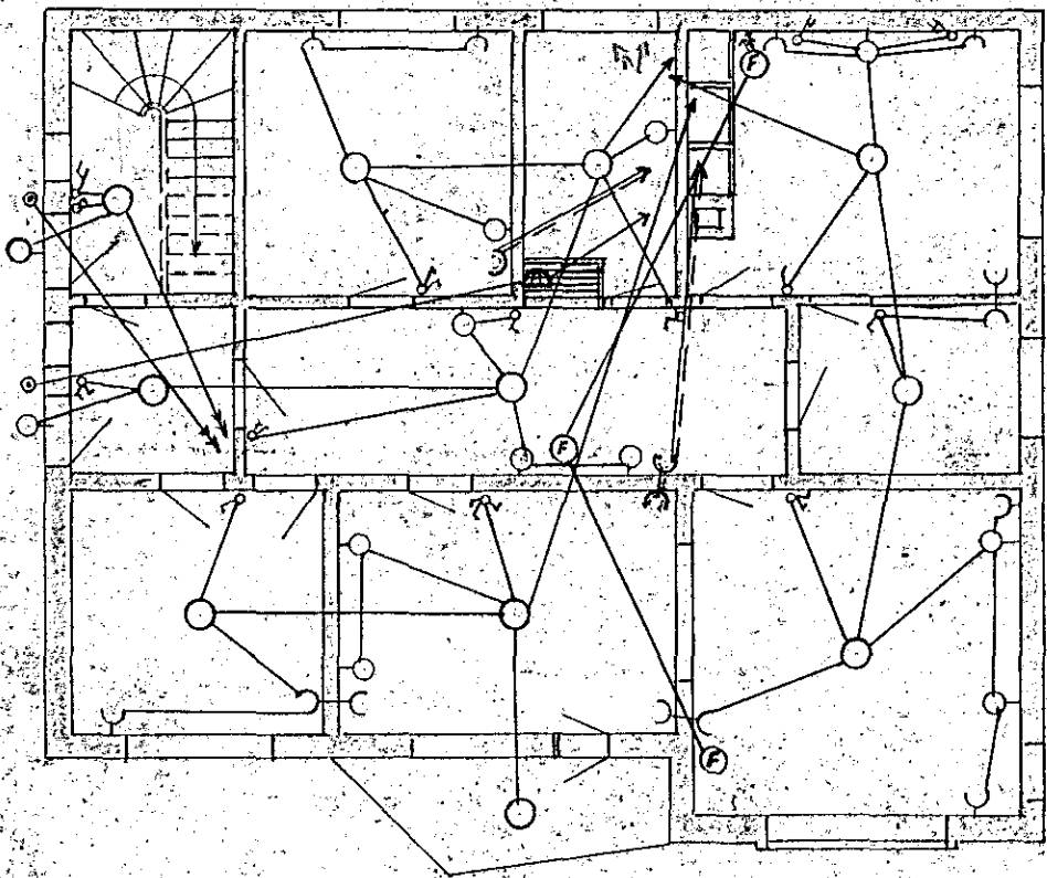
I. hæð
