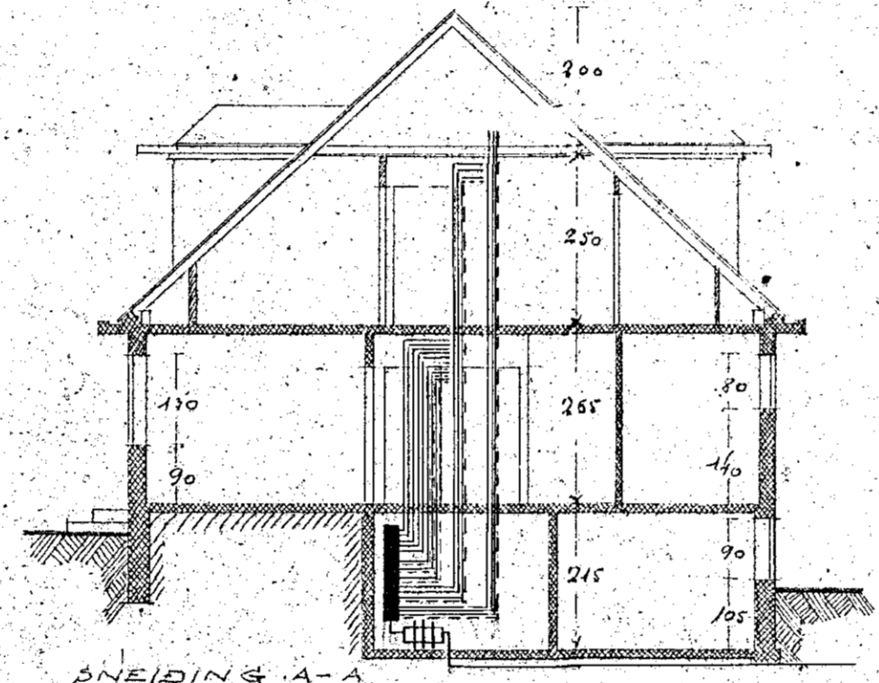
SNEIDING A-A
