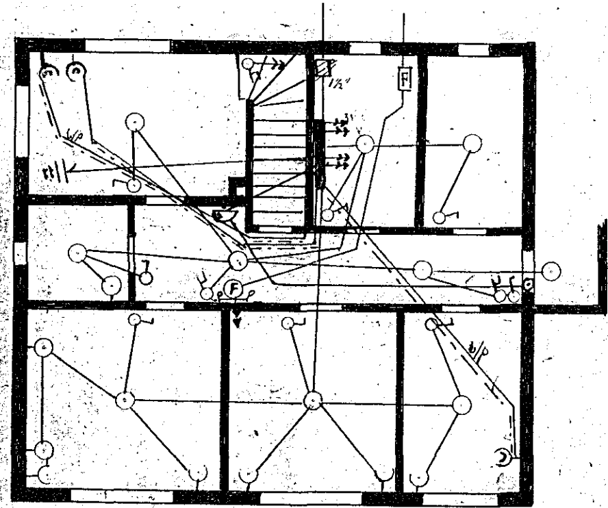
Kjallari
