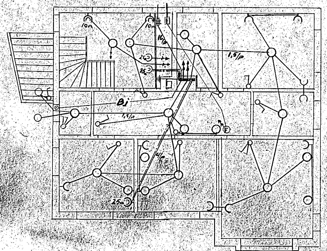
Kjallari
