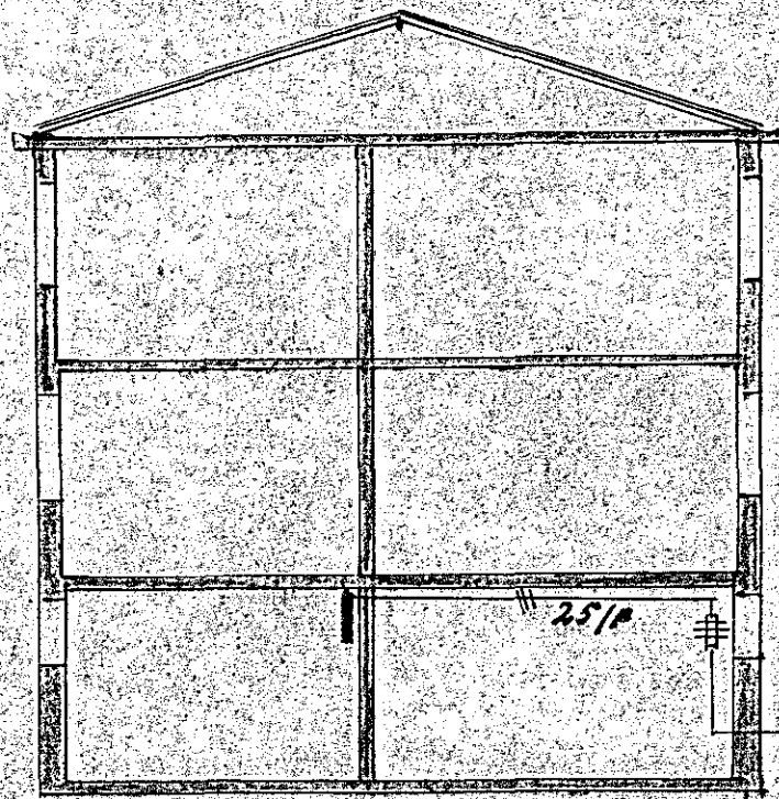
Þverskurður
