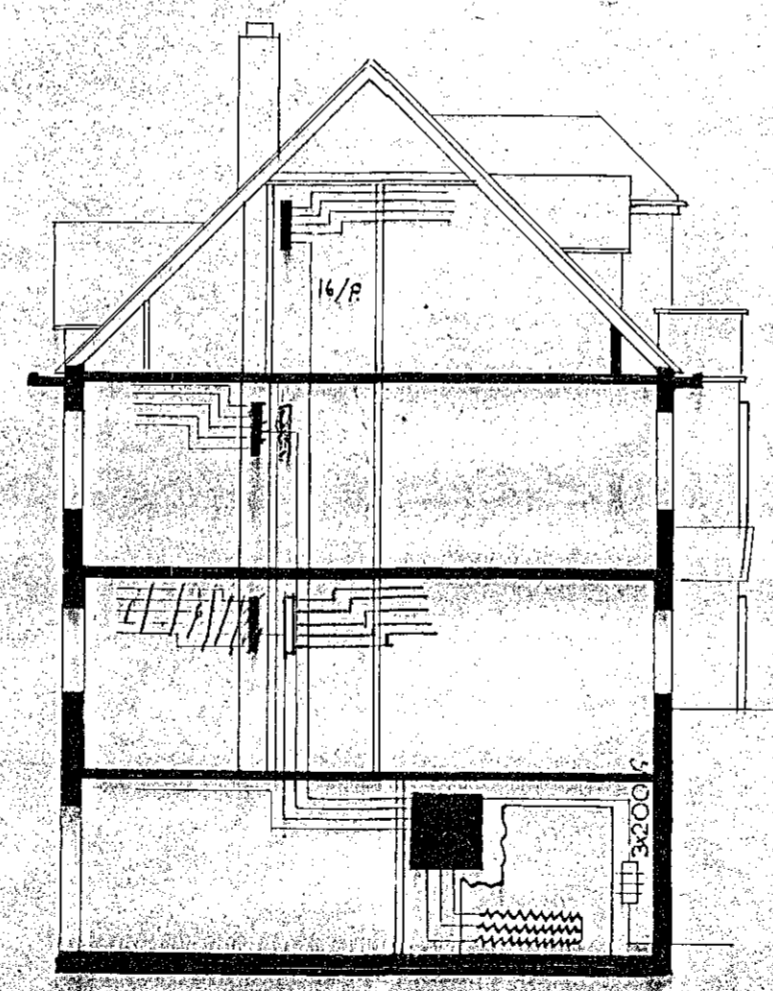
ÞVERSKURÐUR
