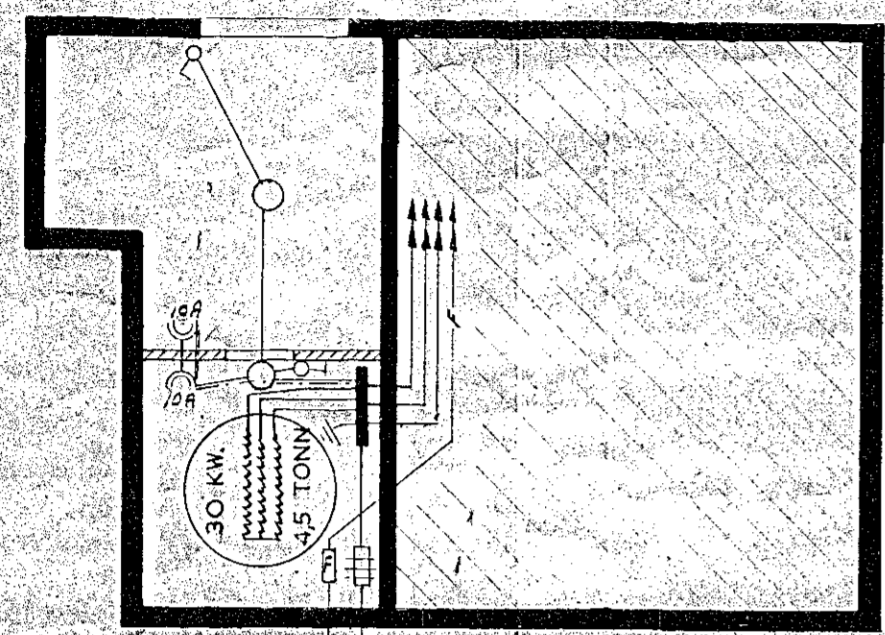
KJALLARI
