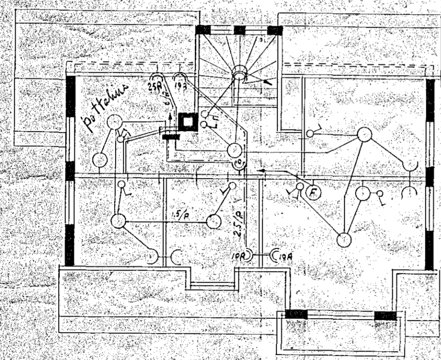
ÞAKHÆÐ
