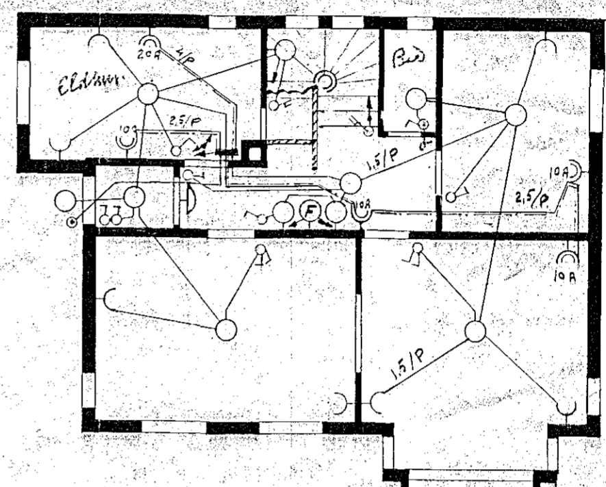
2. HÆÐ
