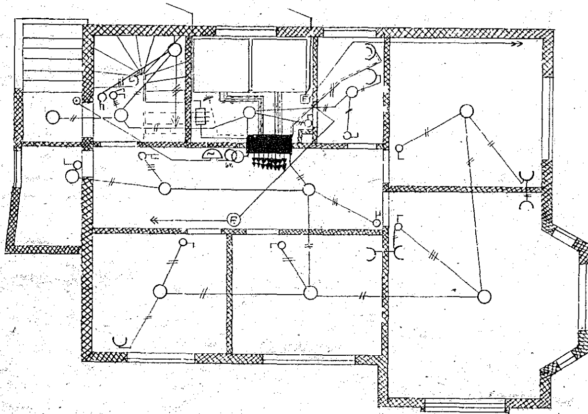
Kjallari.
