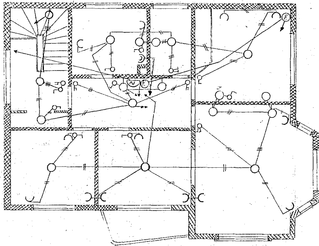
2. hæð.
