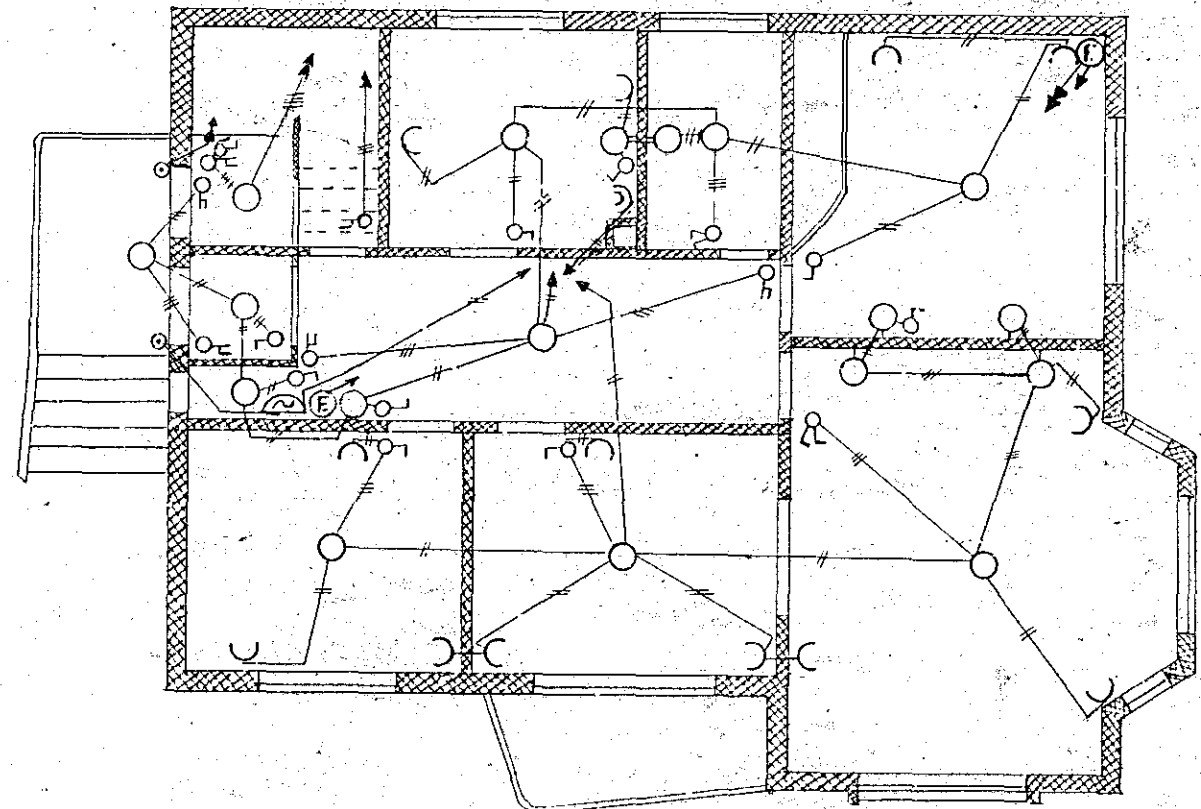
1. hæð.
