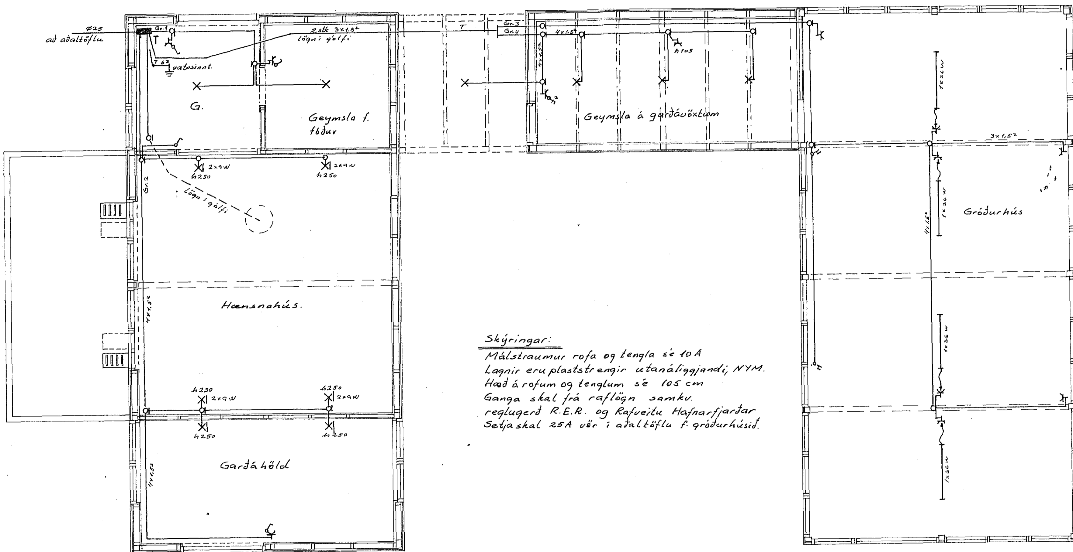
Grunnmund M 1:50
