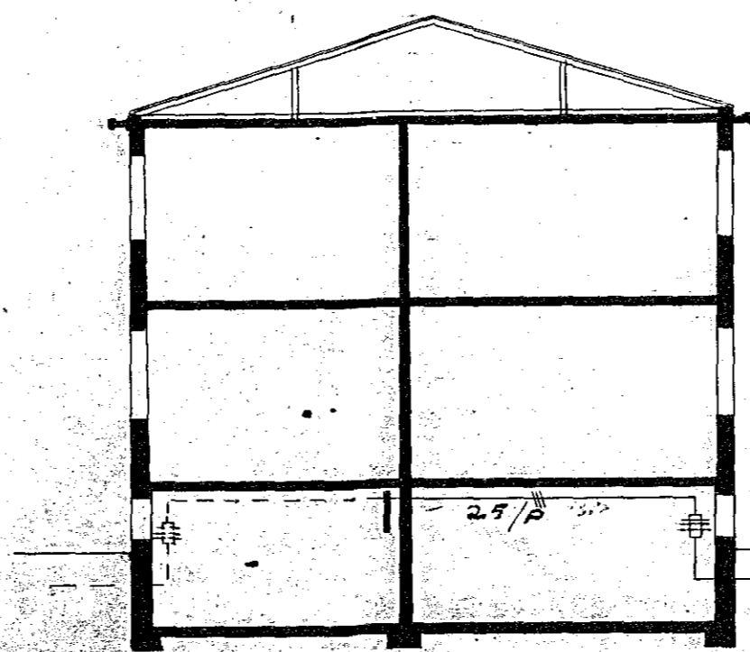
Þverskið
