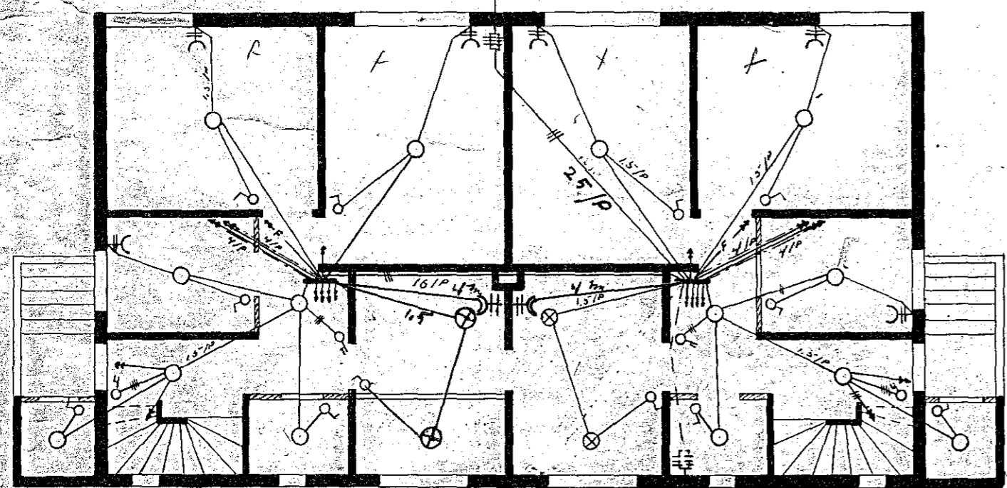
1. hæð
