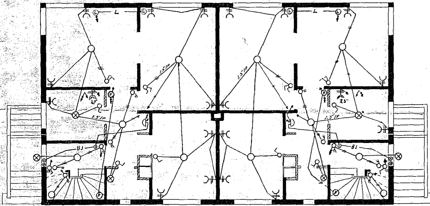
1. hæð
