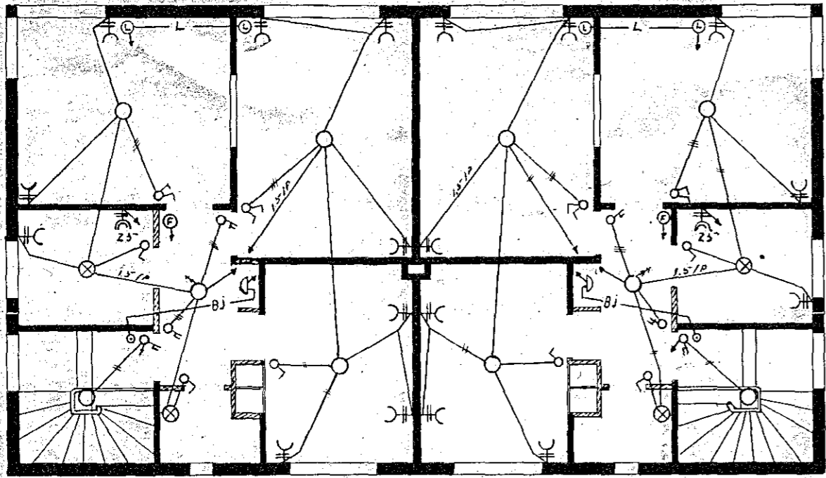
2. hæð
