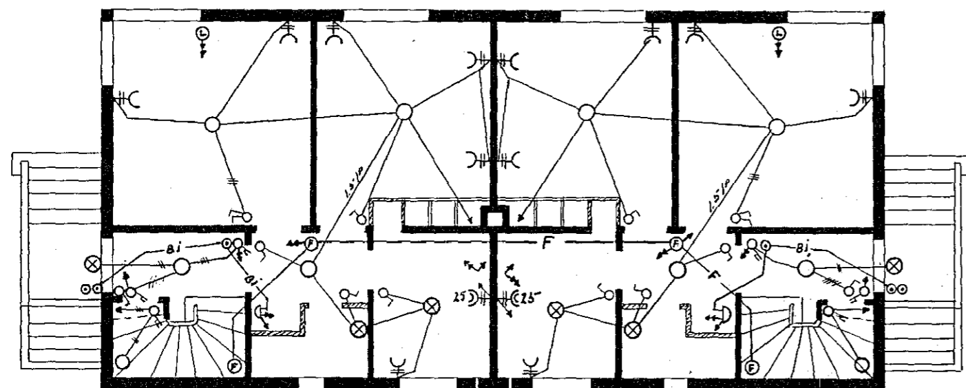
1. hæð
