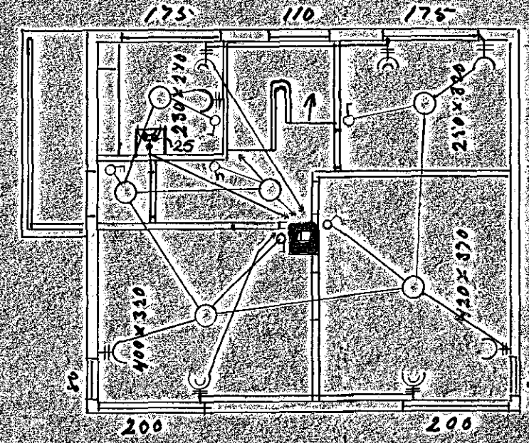
Stofuhæð
