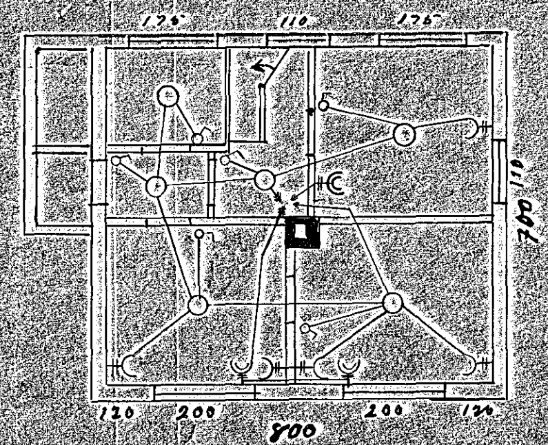
Kjallari
