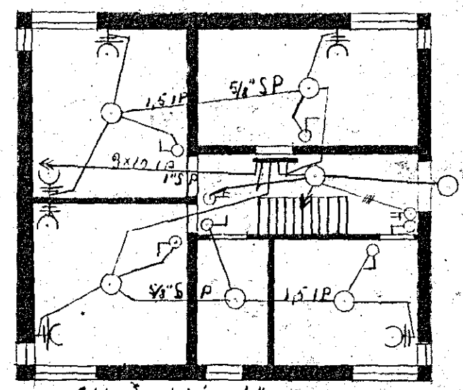
1. hæð ljósabögn
