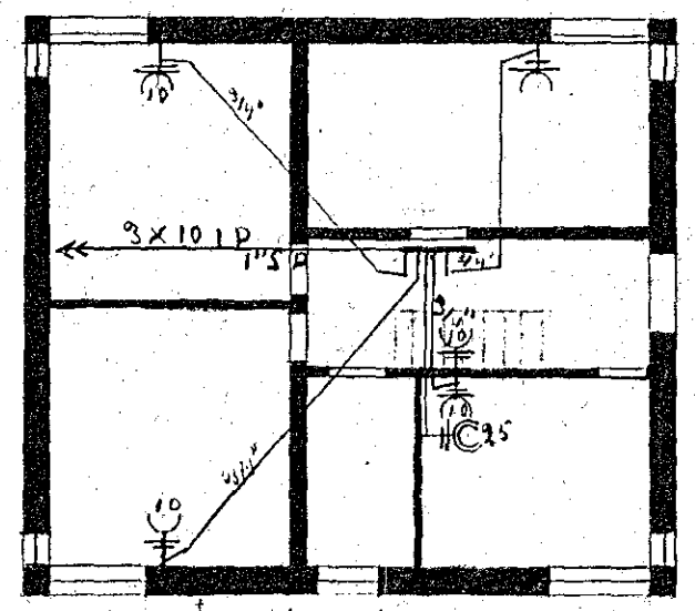
1. hæð hitabögn
