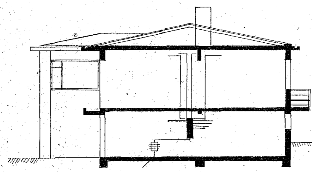
Þverskurður
