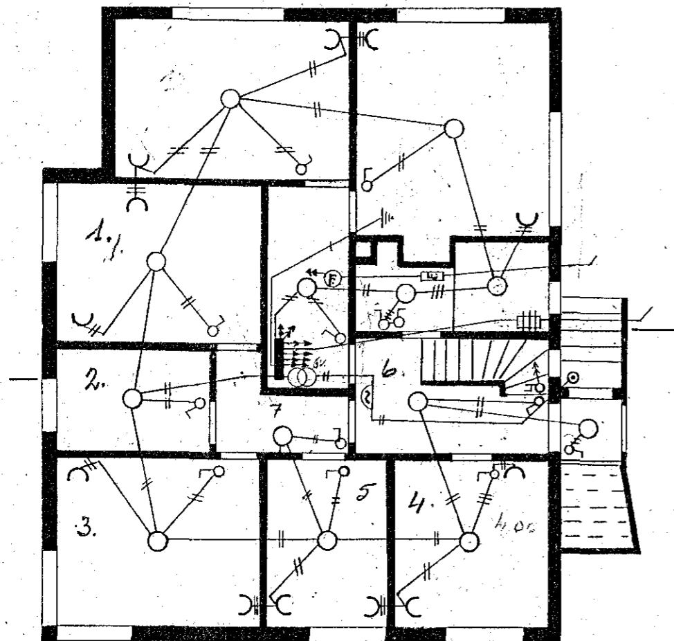
Kjallari.
