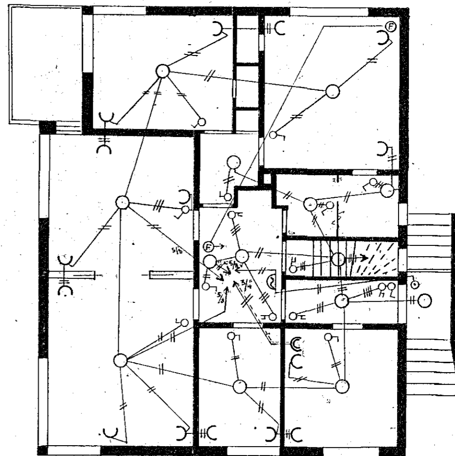
Hæð.
