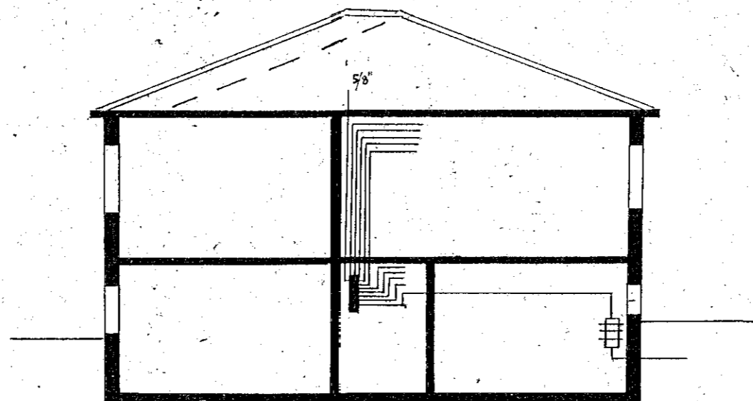
Þverskurður A-A.
