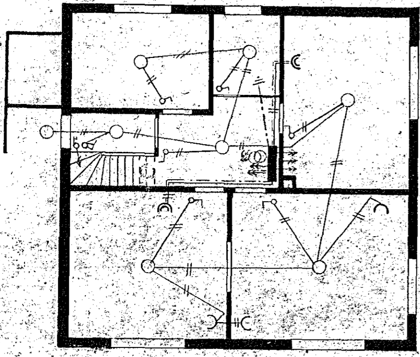
Kjallari.
