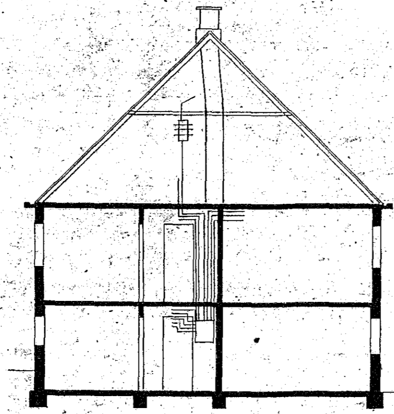
Þverskurður.
