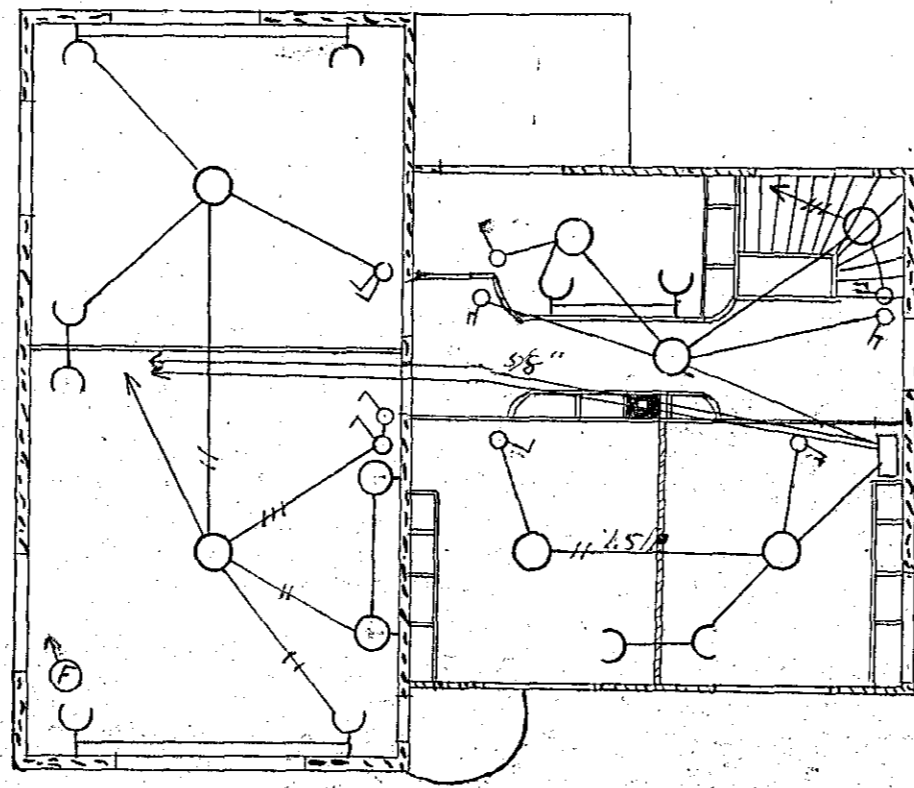
2. Hæð
