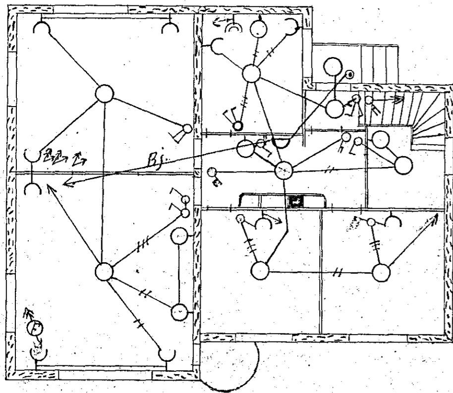
1. Hæð
