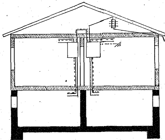
Þverskurður.
