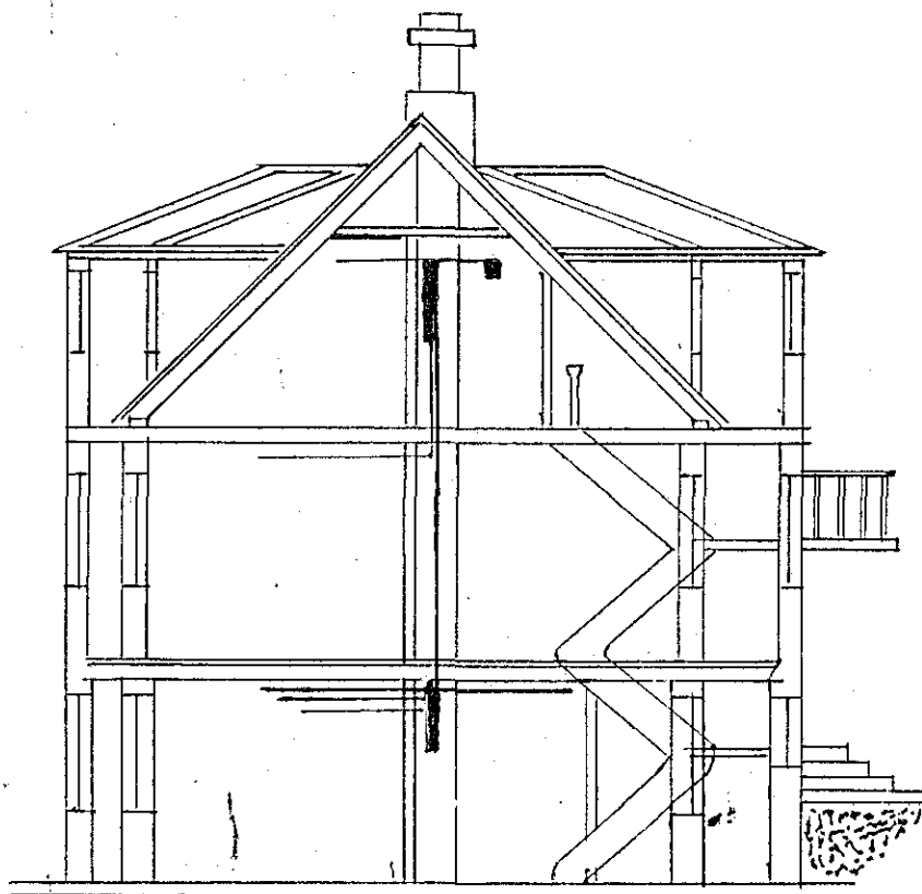
Skurður
