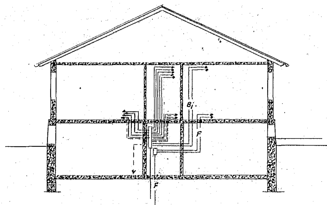
Þverskurður
